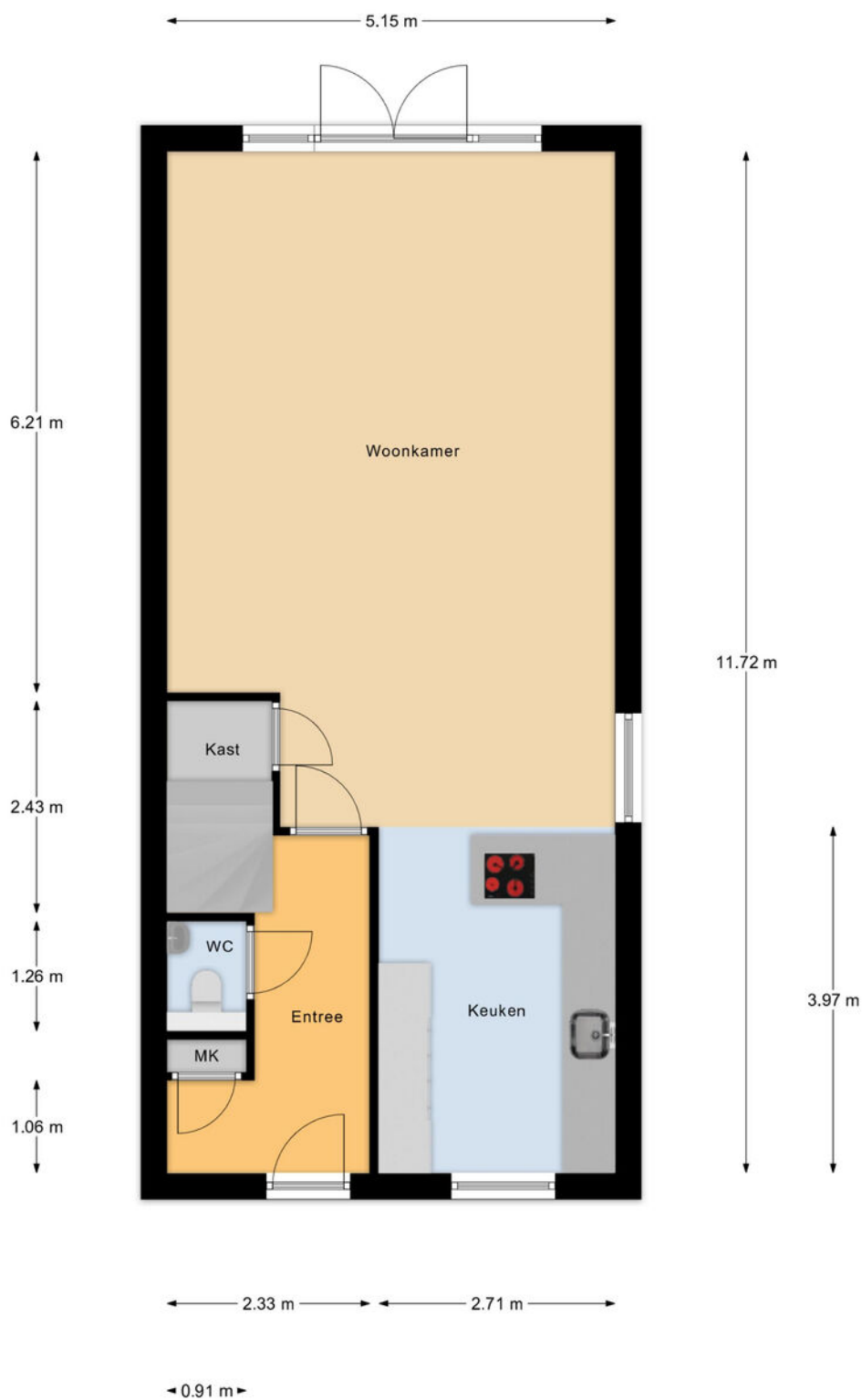
Begane Grond
