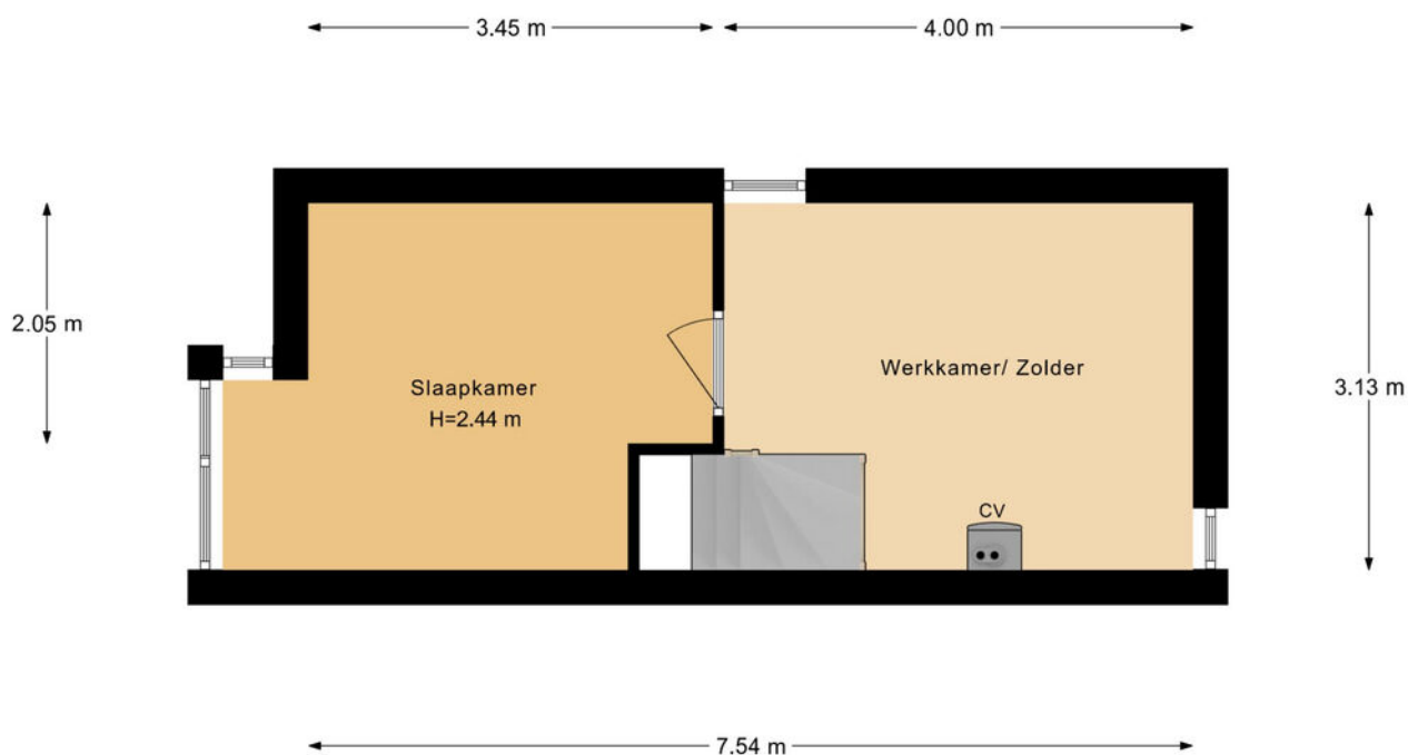
2e Verdieping
