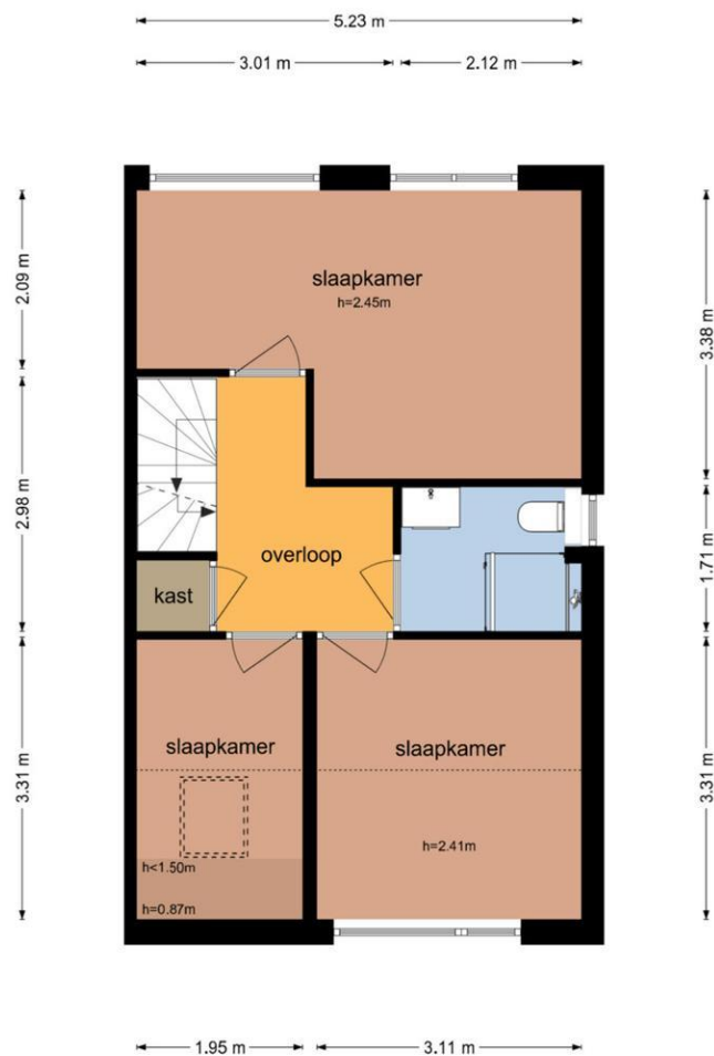
Gasthuisbouwing 19 - Rheden Eerste Verdieping
