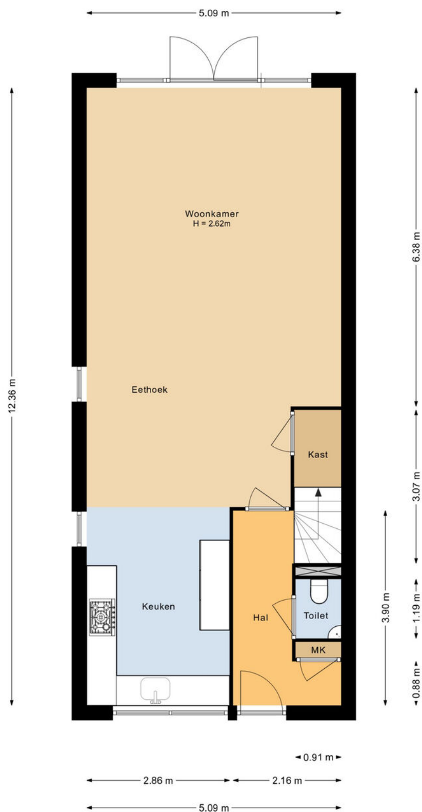
Begane grond Piet Heinstraat 22 Lisse
