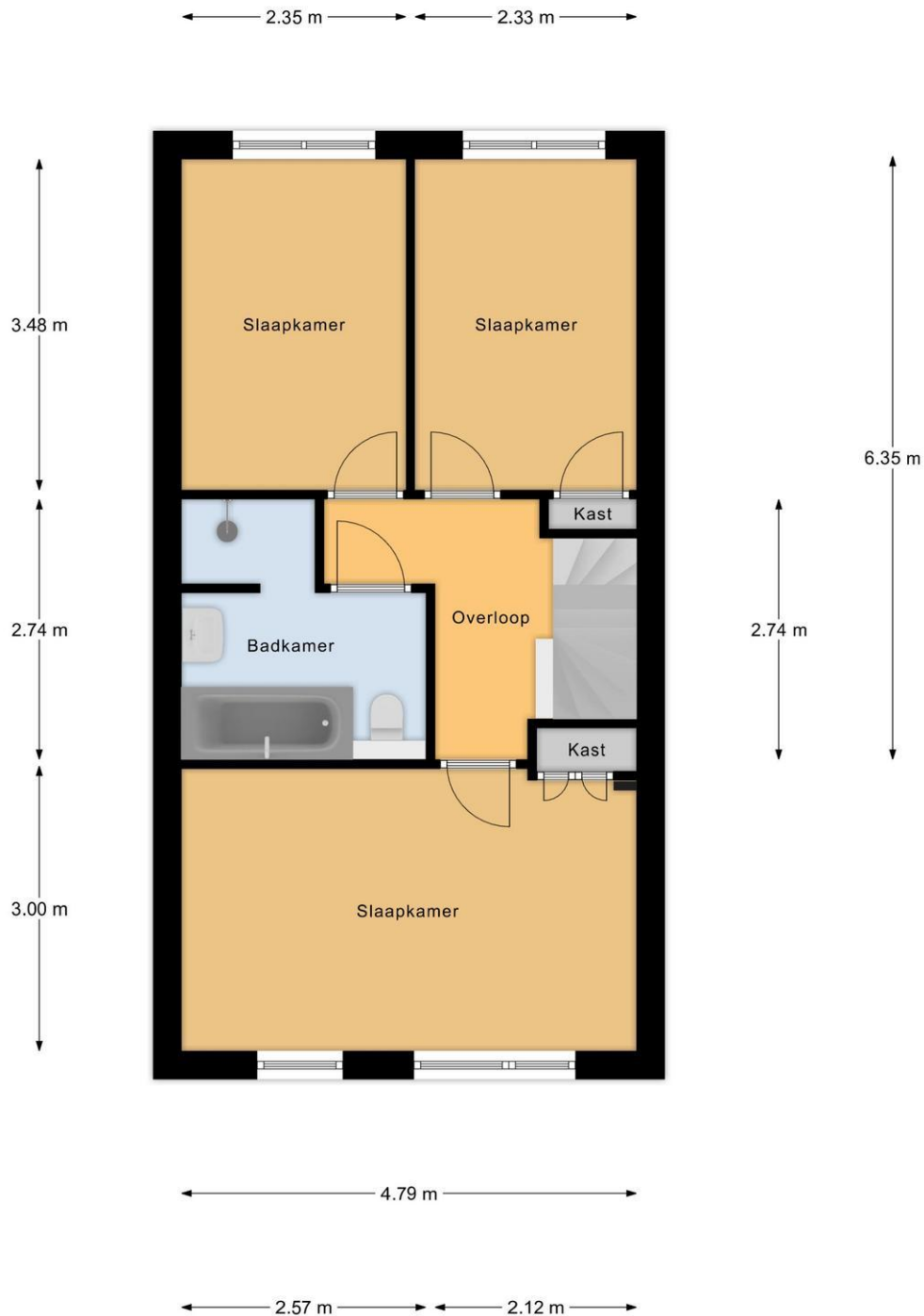
1e Verdieping
