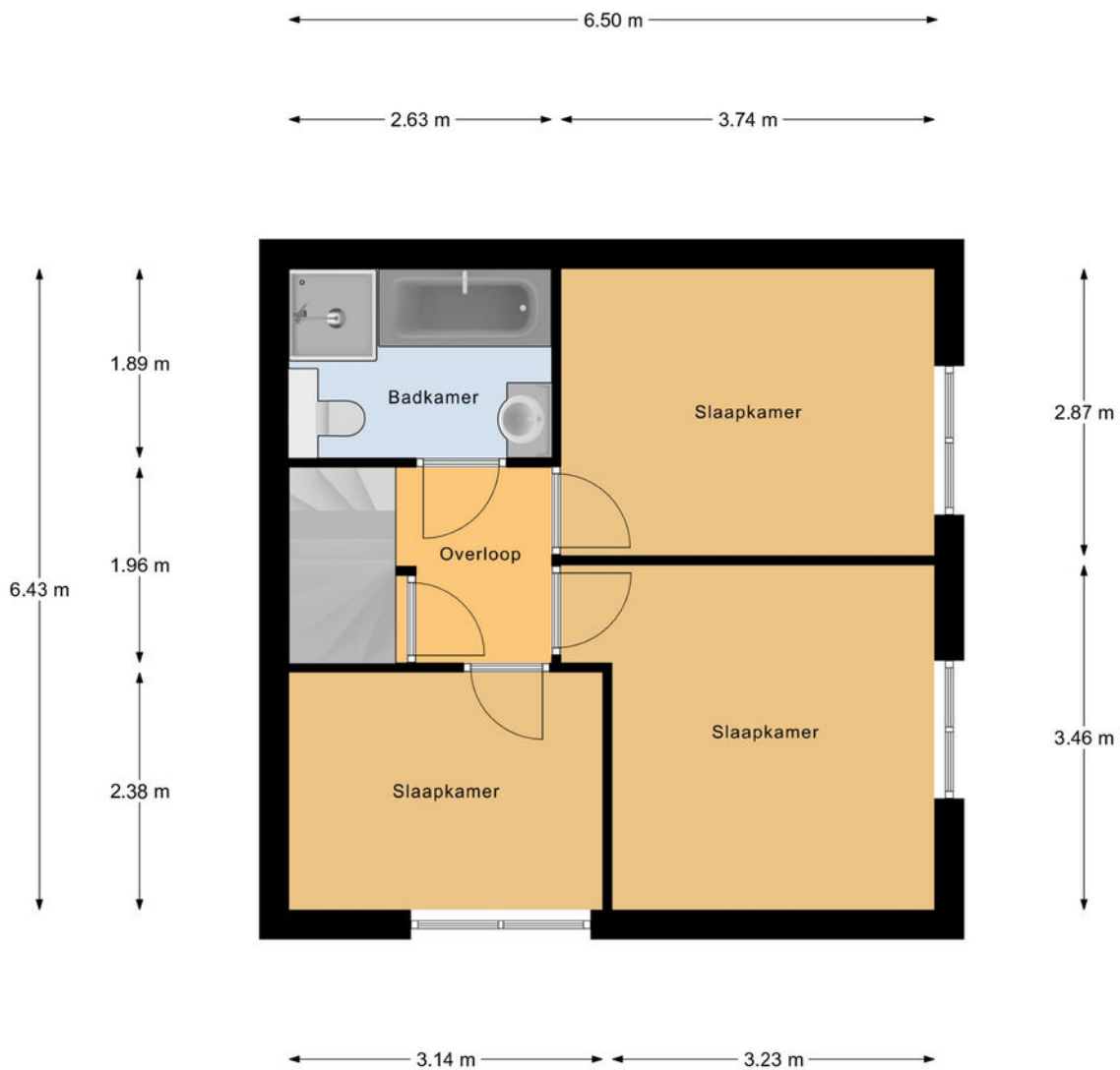
1e Verdieping
