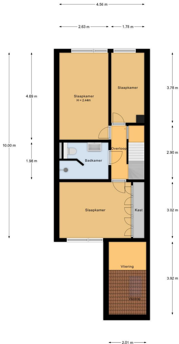
1e Verdieping
