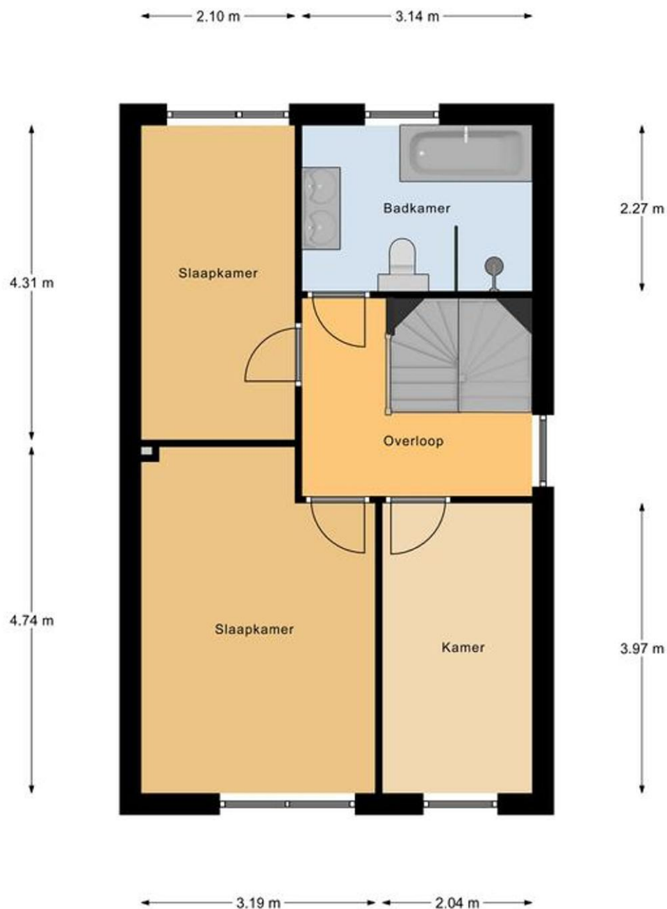
1e Verdieping
