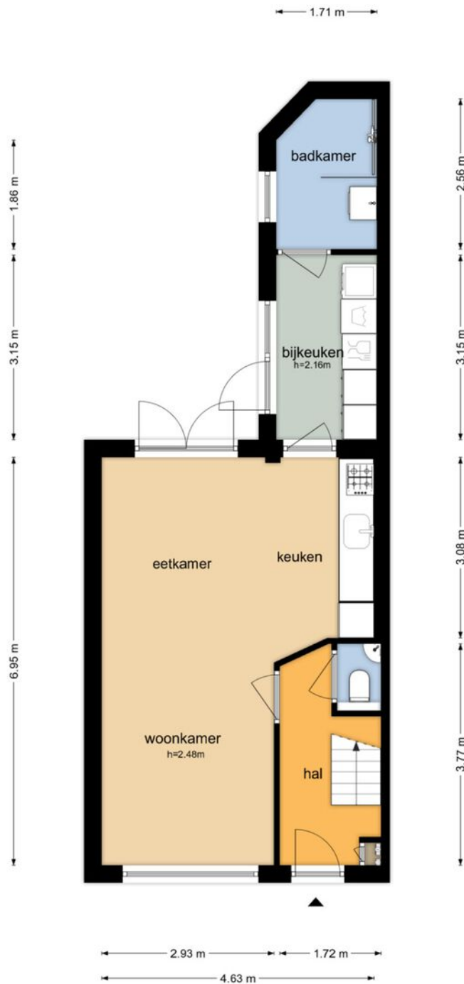
Burgemeester Schoutsenstraat 13 - Medemblik Begane Grond
