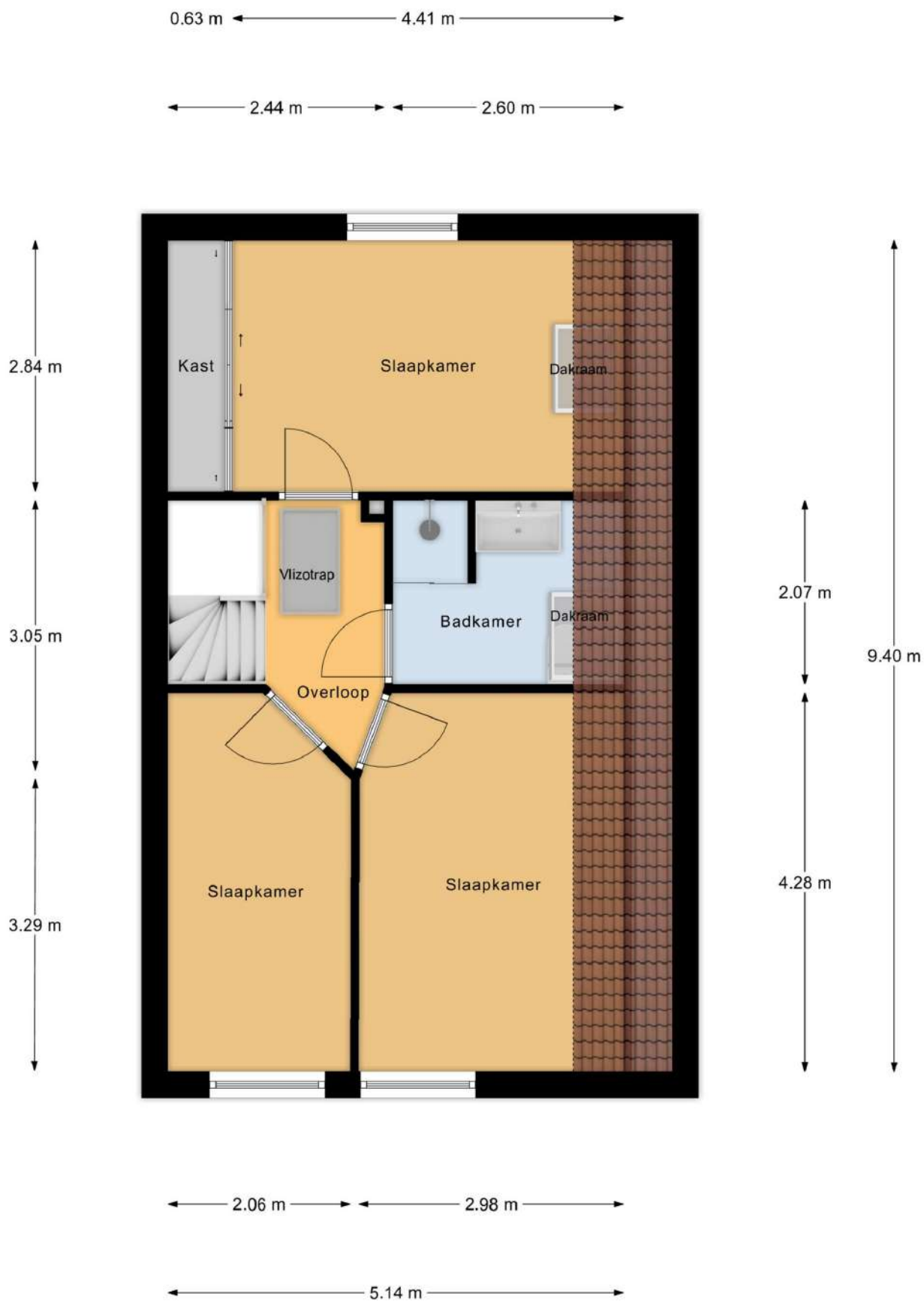
1e Verdieping
