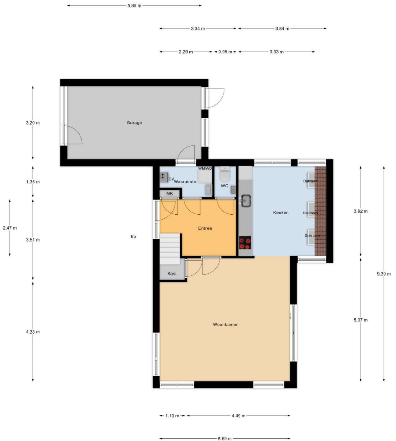
Begane Grond
