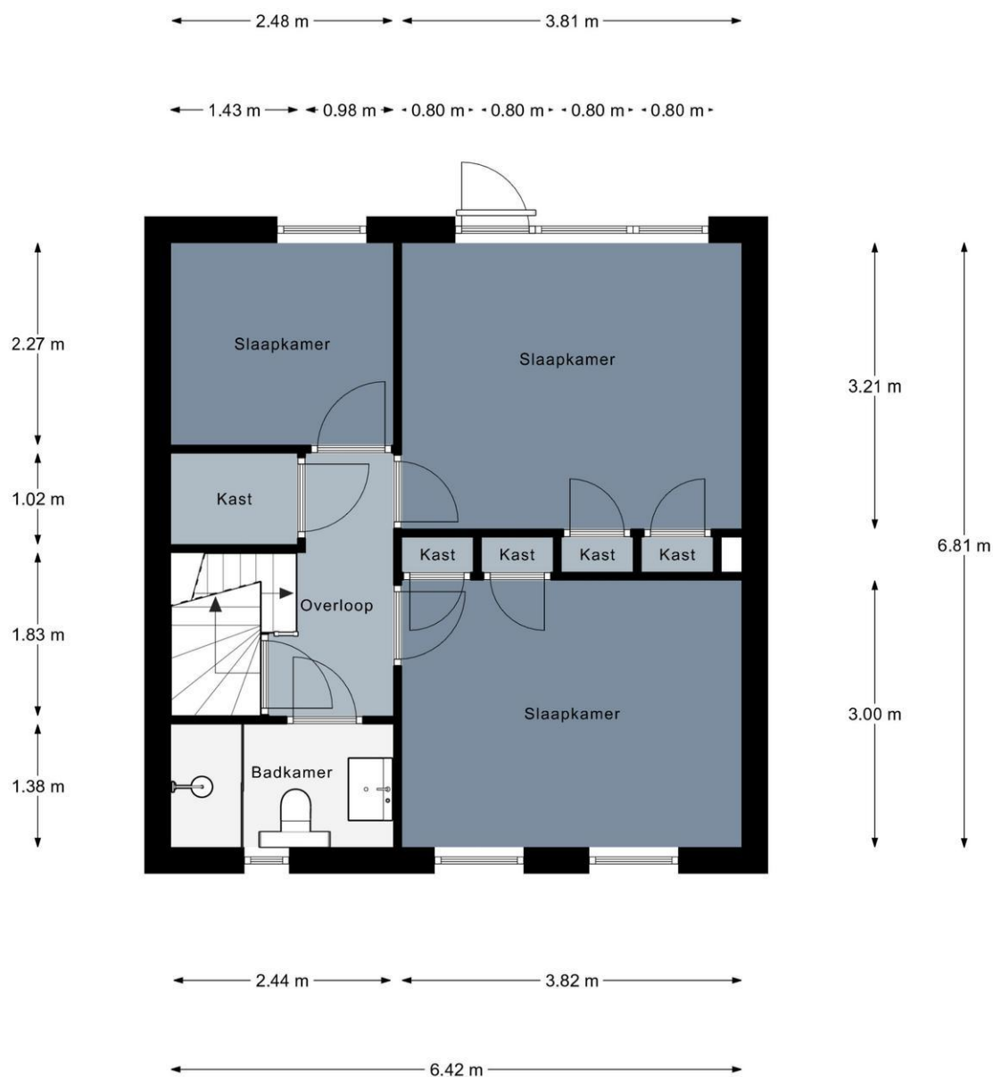
1e Verdieping
