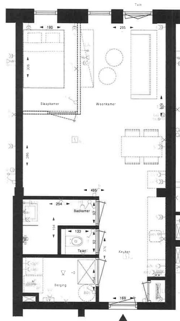
25F1 Begane Grond 1 : 50
