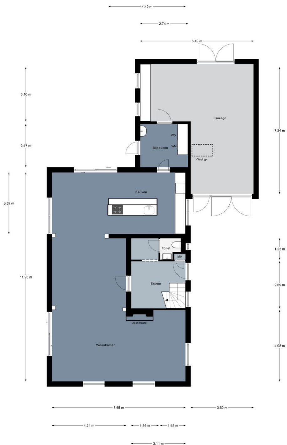
Begane Grond
