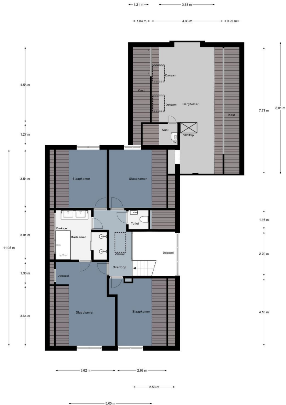
1e Verdieping
