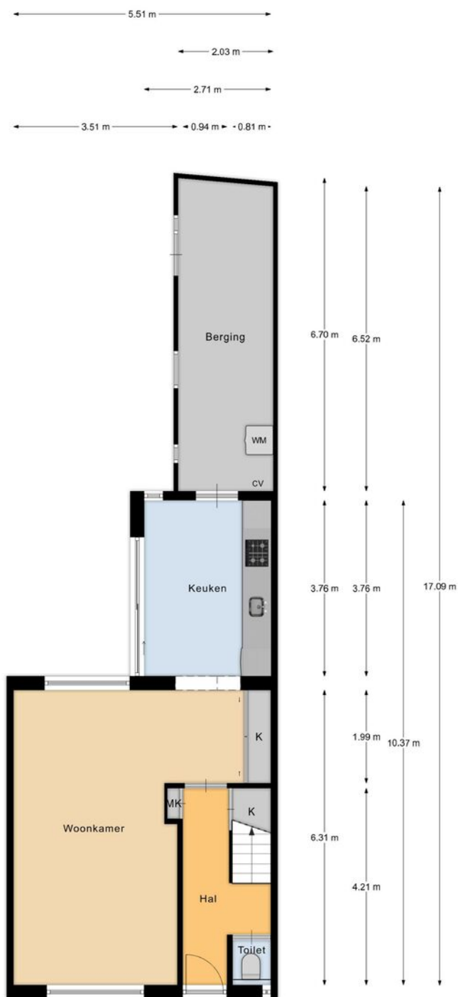
Begane grond
