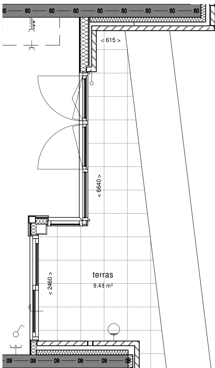
Zuidgevel Bouwnrs.: 01.09
