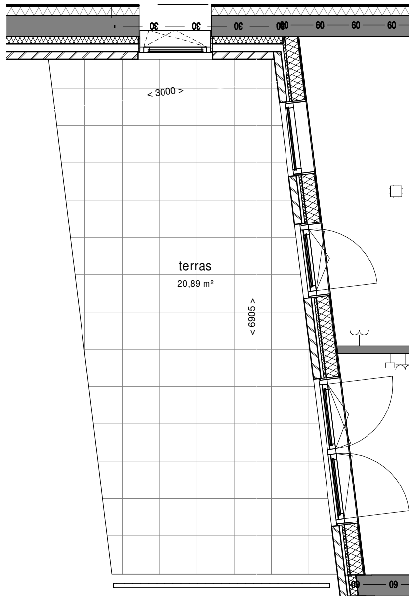
Noordgevel Bouwnrs.: 01.09
