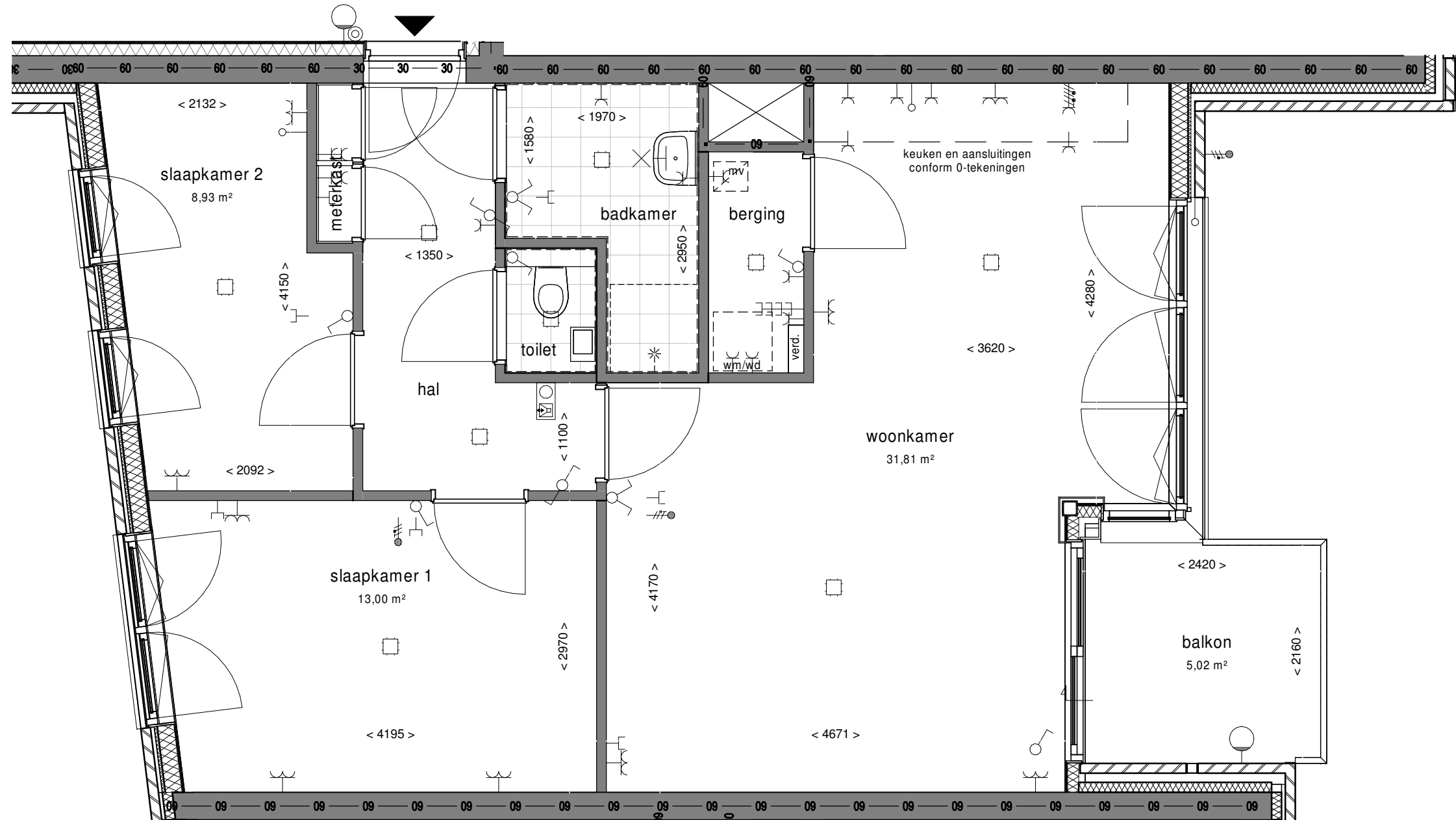
Noordgevel Bouwnrs.: 02.10/03.10/04.10/05.05
