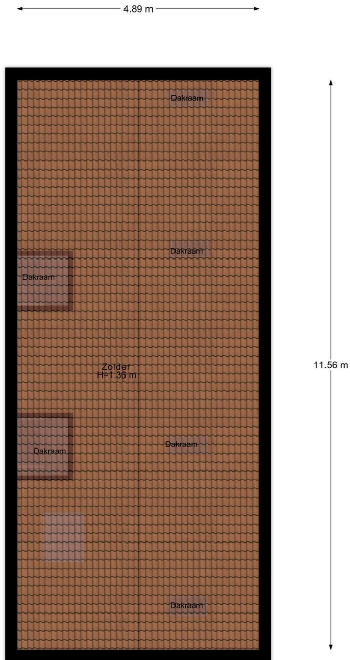
2e Verdieping
