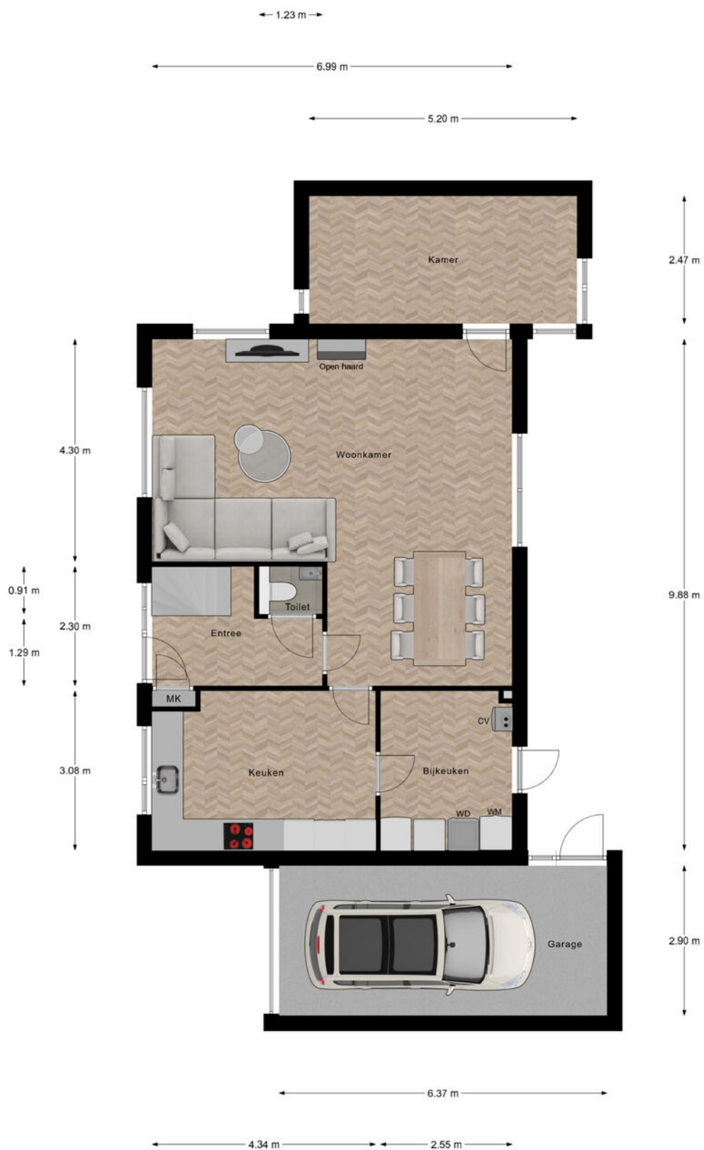
Begane Grond
