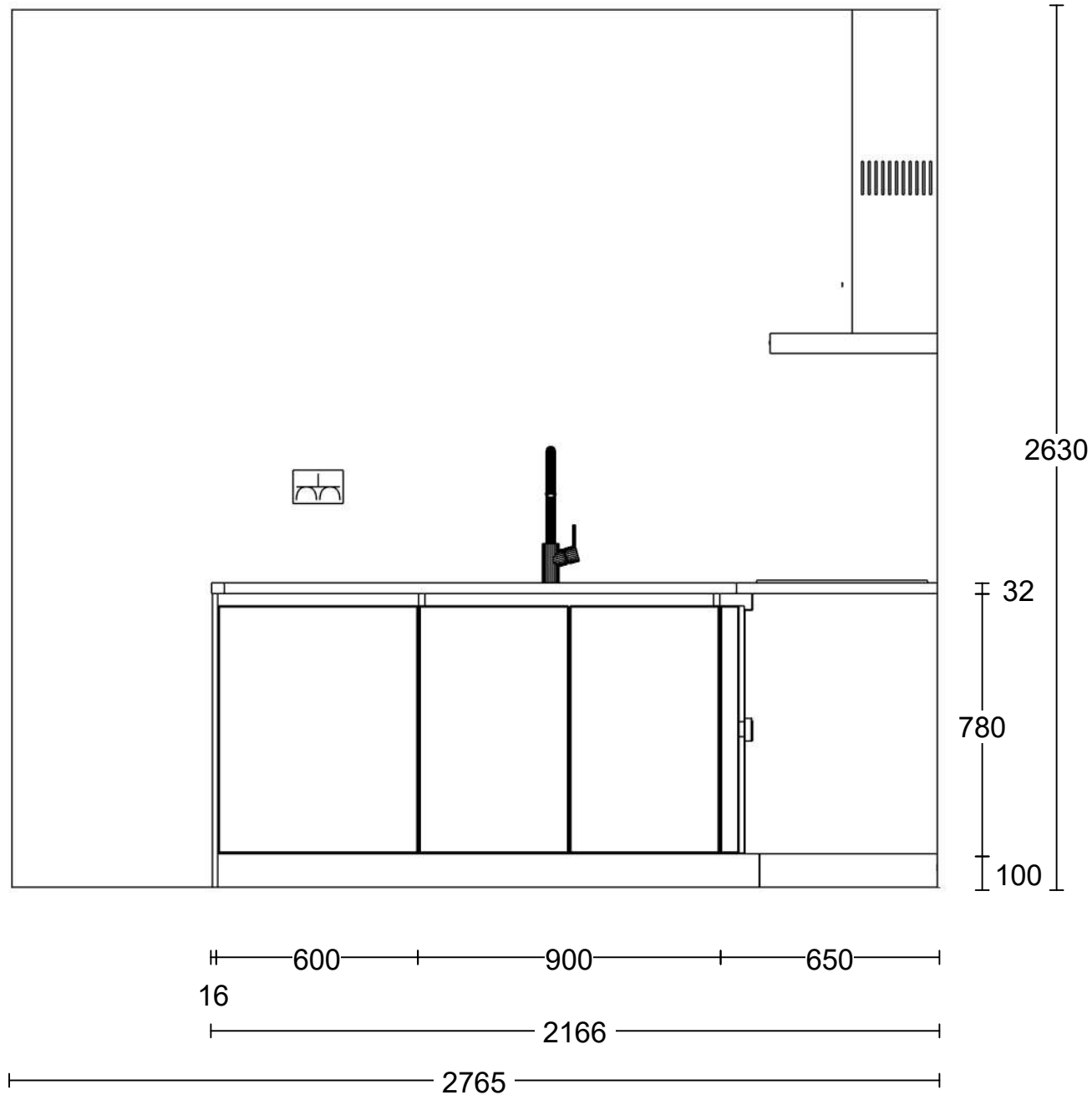
Vooraanzicht wand 1
