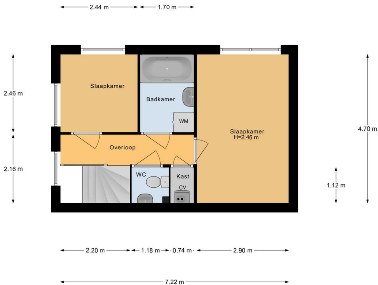
2e Verdieping
