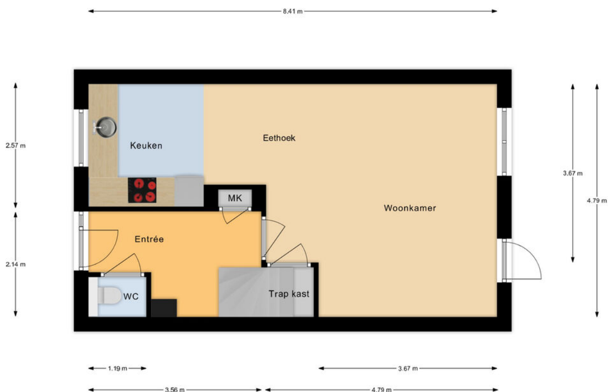
Begane Grond
