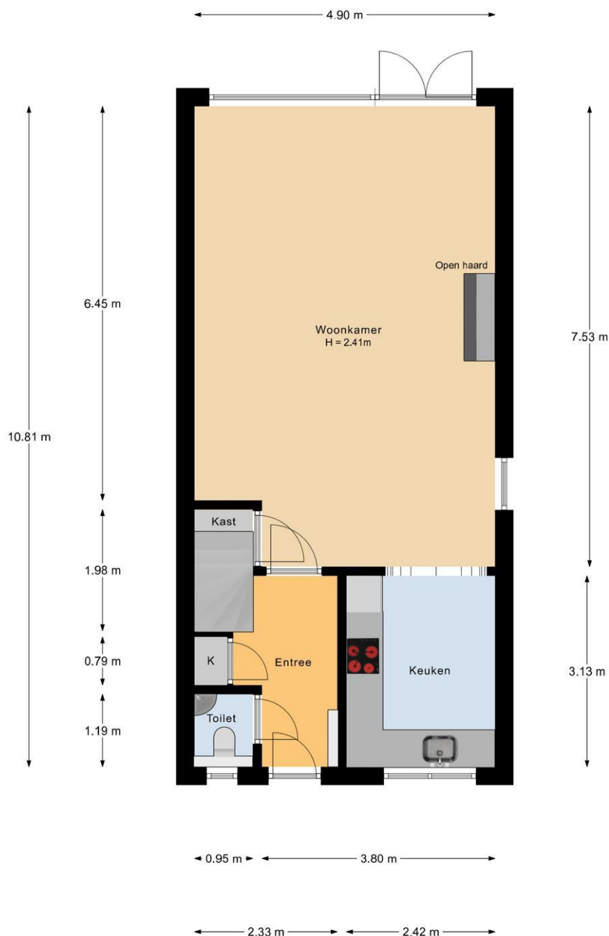
Begane Grond
