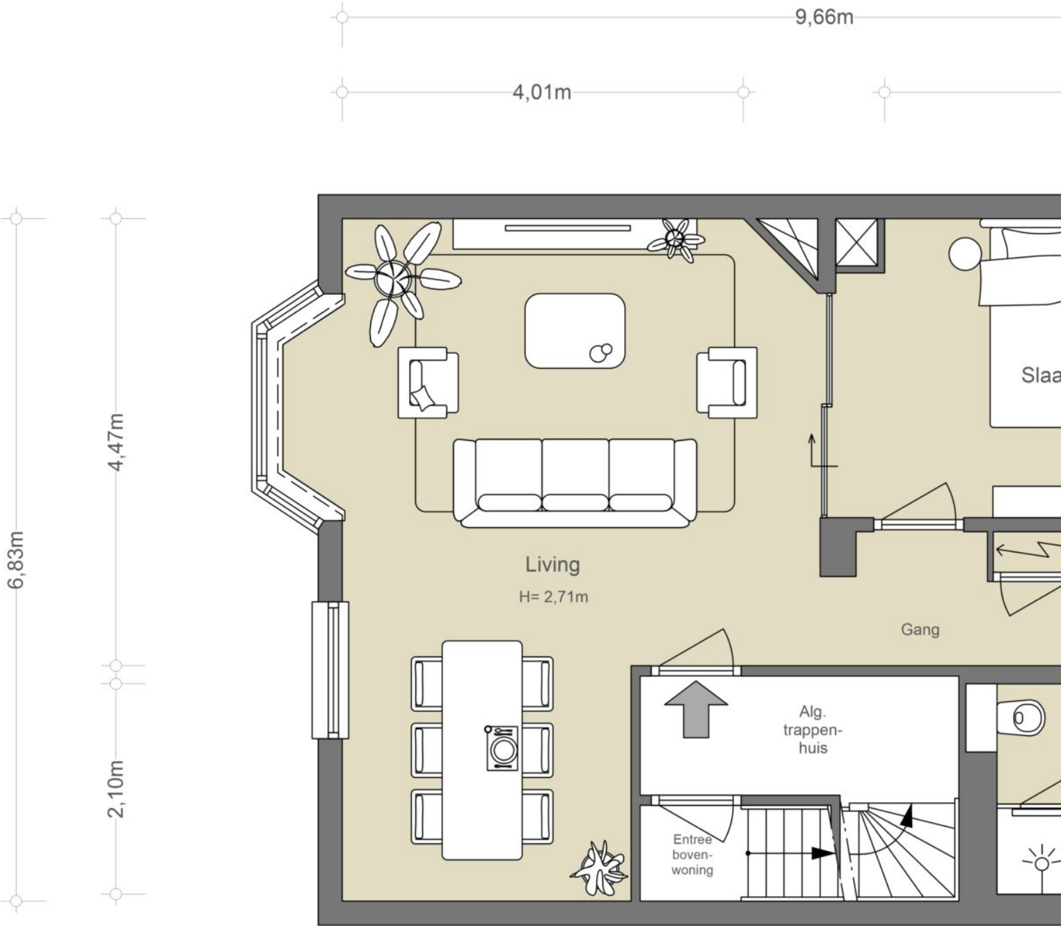
DERDE VERDIEPING
