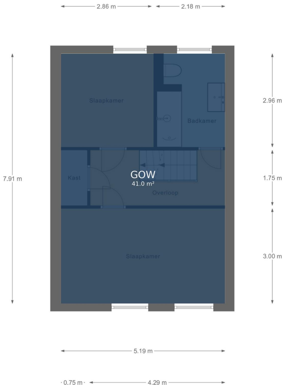
1e Verdieping
