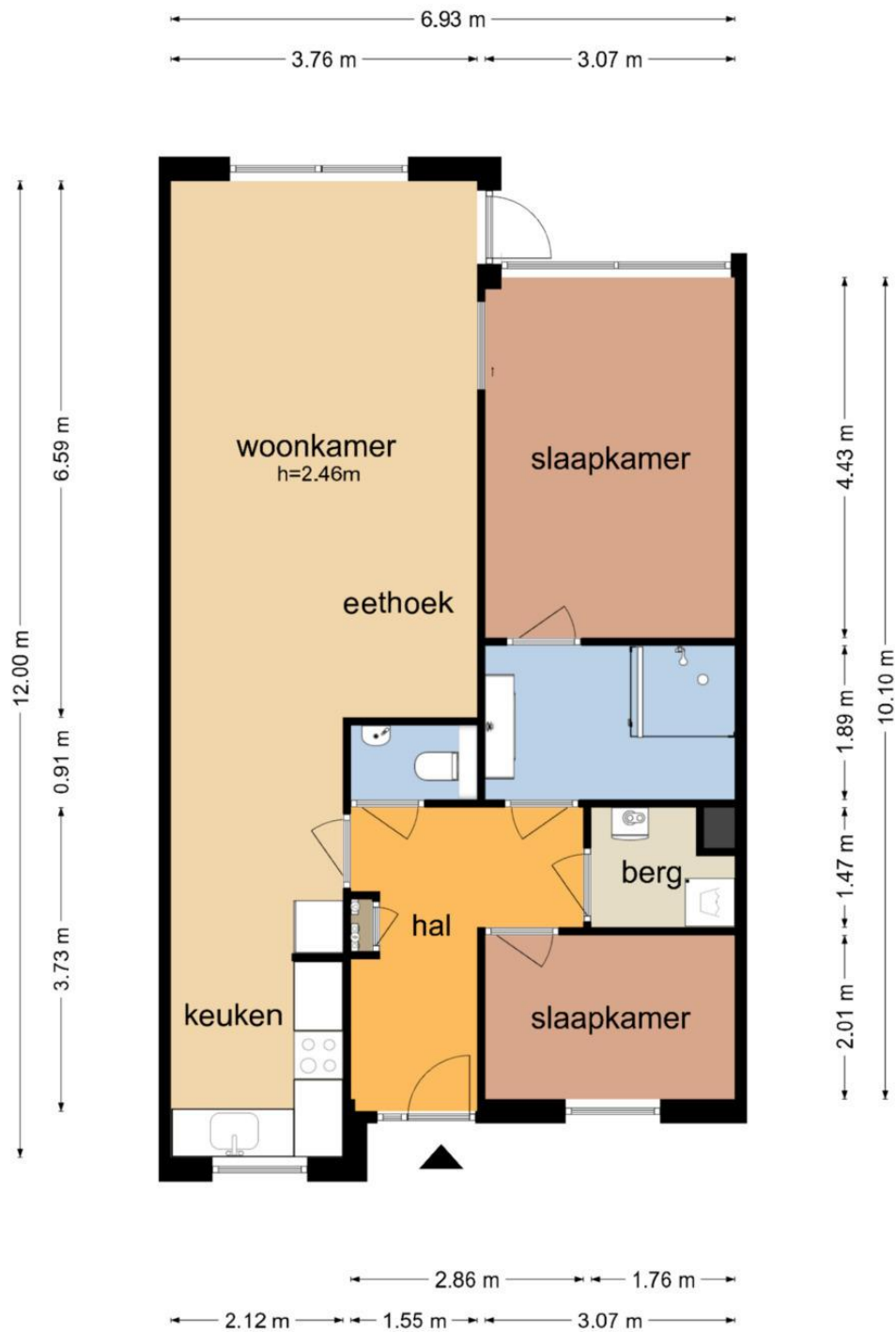
Kantbeugel 65 - De Goorn Begane Grond
