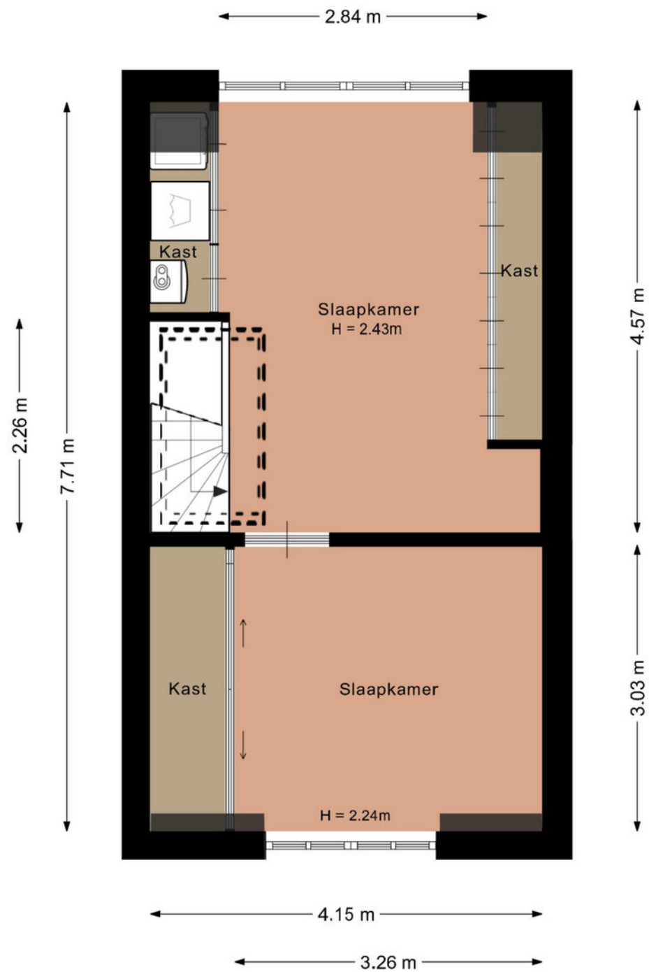
Griftstraat 62, Utrecht Tweede verdieping
