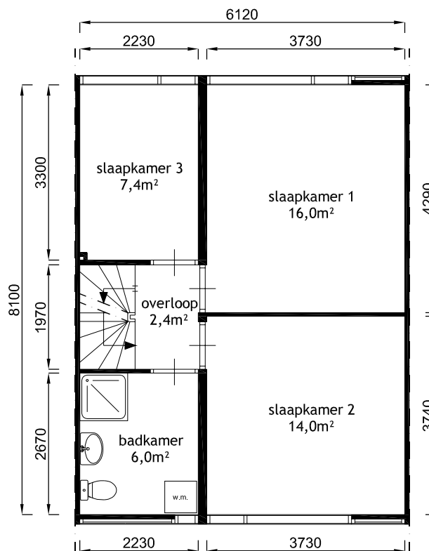
1e verdieping
