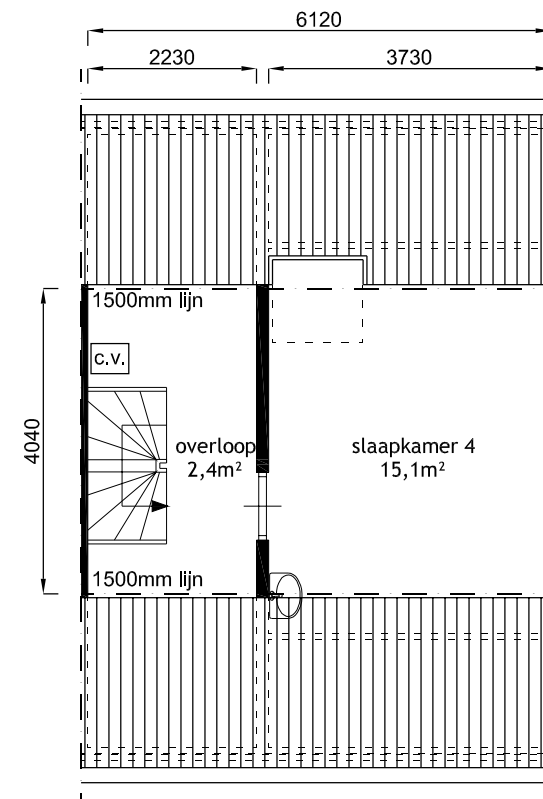
2e verdieping
