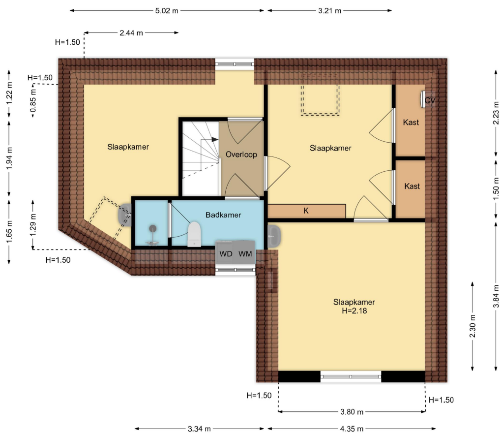
1e Verdieping Meerweg 17, Bennebroek R.M. Vastgoedpresentatie| Aan deze plattegrond kunnen geen rechten worden ontleend
