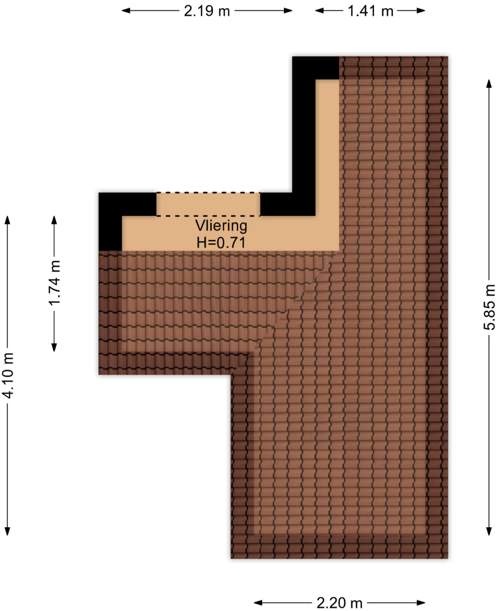
Vliering Meerweg 17, Bennebroek R.M. Vastgoedpresentatie| Aan deze plattegrond kunnen geen rechten worden ontleend
