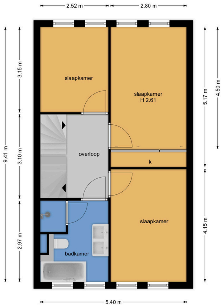
1e verdieping
