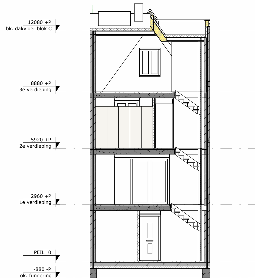
DWARSDOORSNEDE
