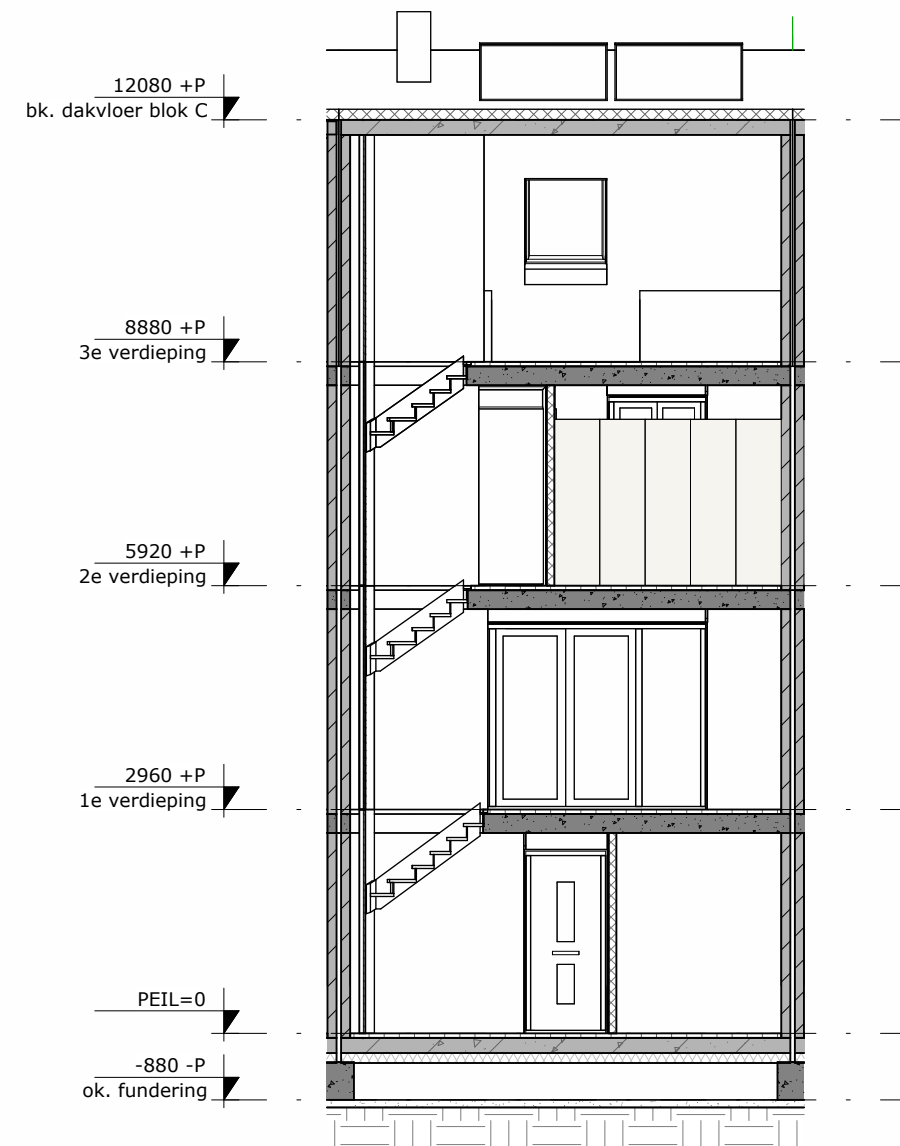
DWARSDOORSNEDE
