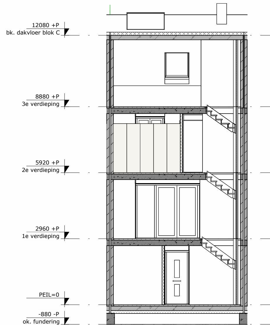
DWARSDOORSNEDE
