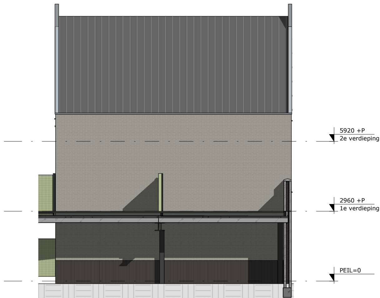
ZIJGEVEL
