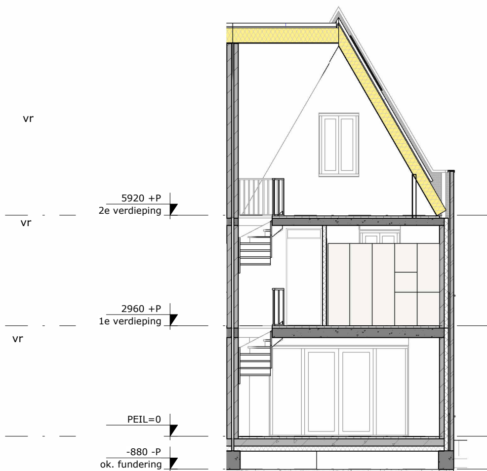
DWARSDOORSNEDE
