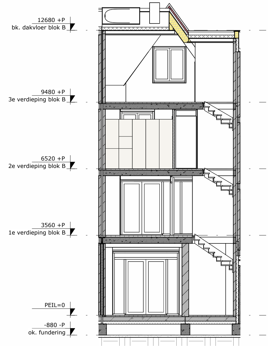
DWARSDOORSNEDE
