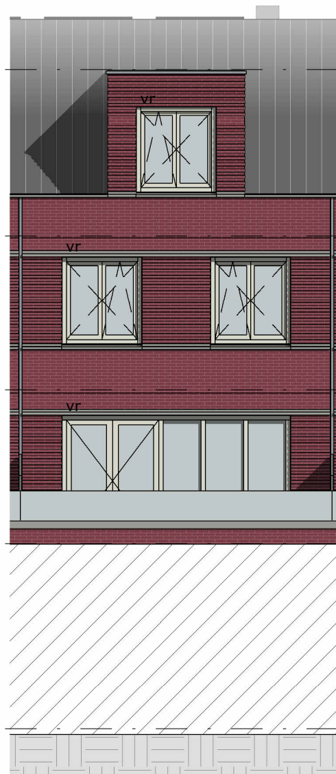
ACHTERGEVEL IJsselmeerzijde noord
