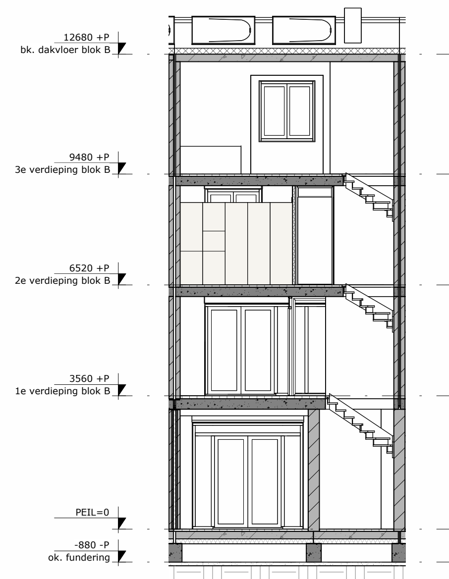
DWARSDOORSNEDE
