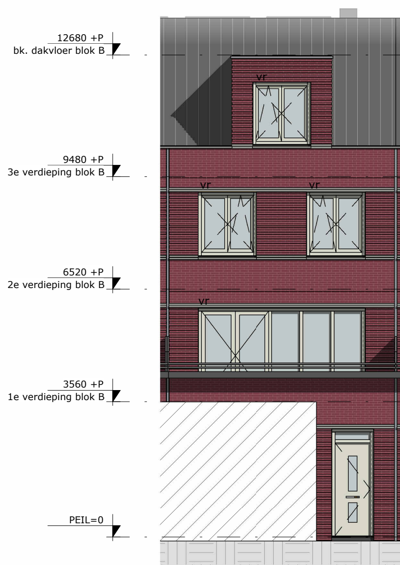
VOORGEVEL Stadsplein zuid
