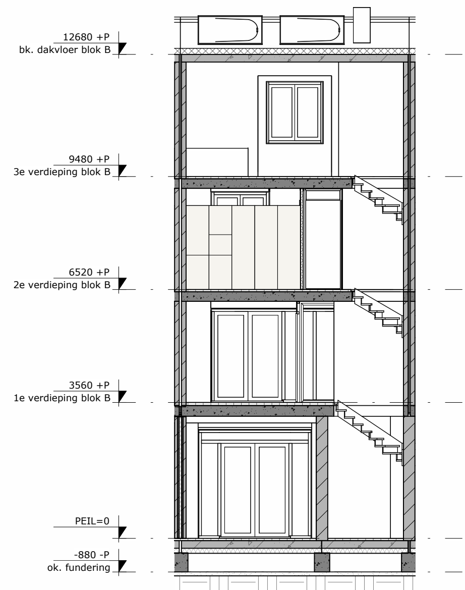
DWARSDOORSNEDE
