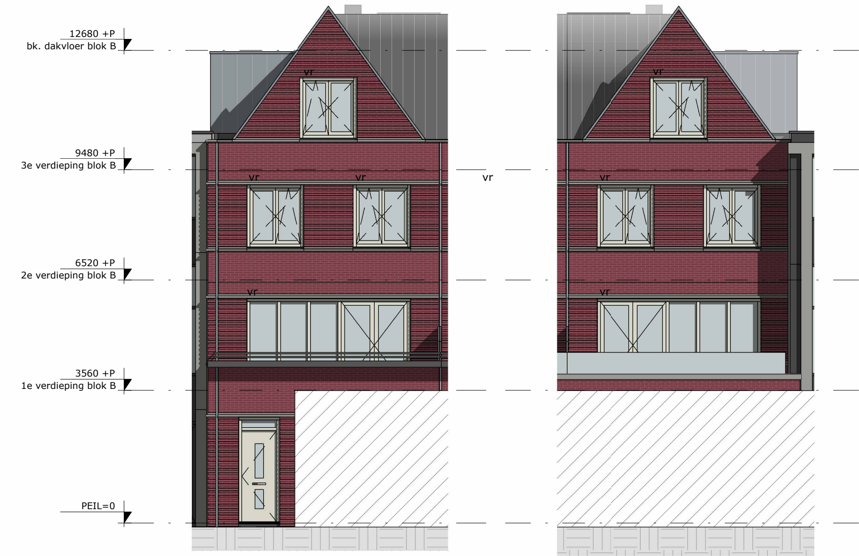
VOORGEVEL Stadsplein zuid
