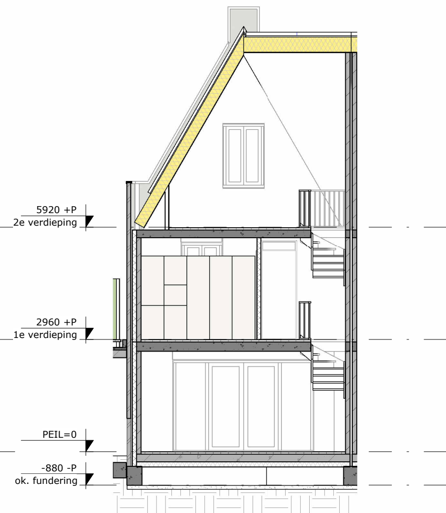
DWARSDOORSNEDE
