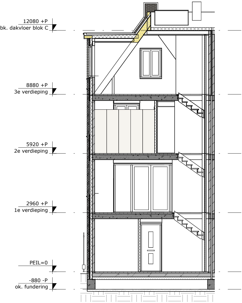
DWARSDOORSNEDE
