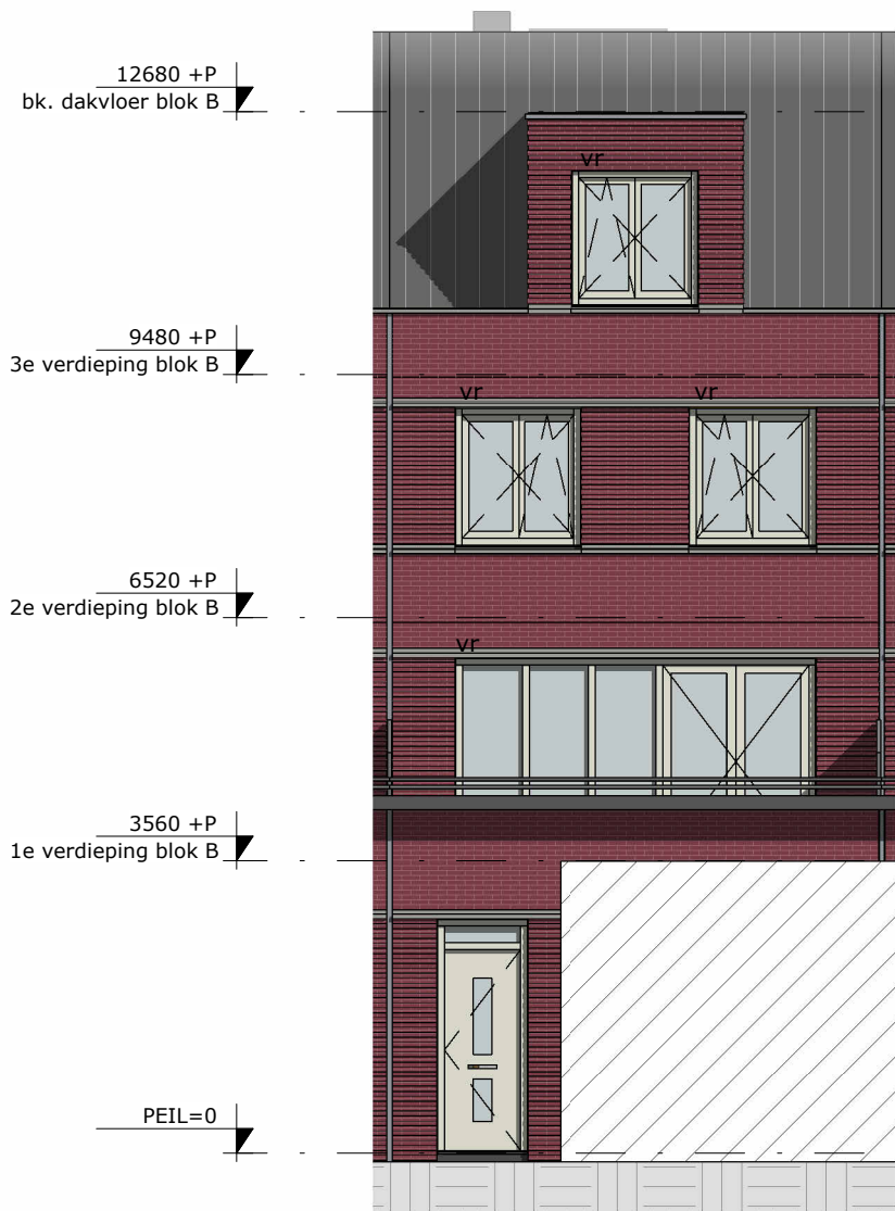
VOORGEVEL Stadsplein zuid
