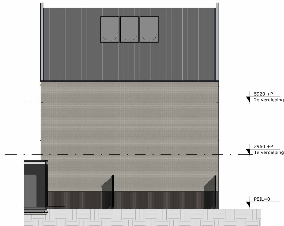
ZIJGEVEL
