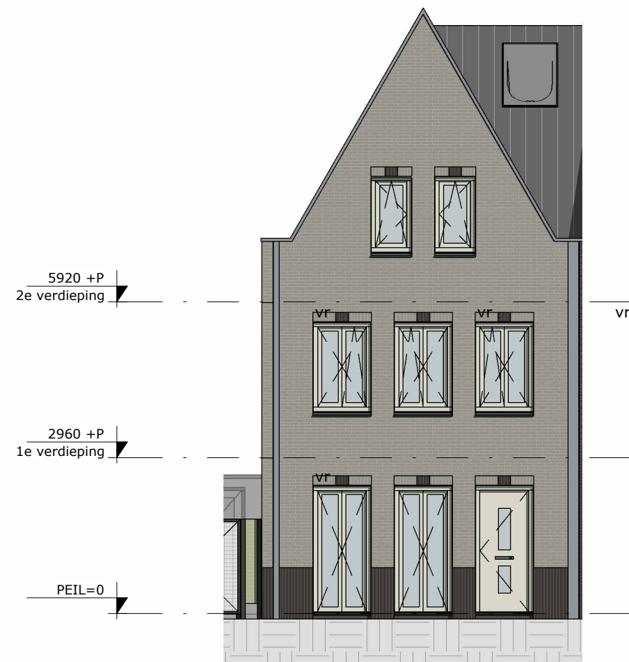
VOORGEVEL
