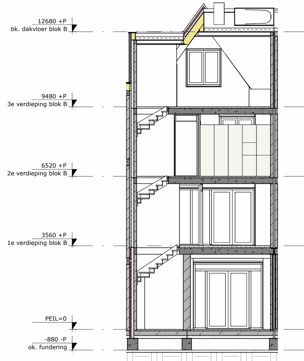
DWARSDOORSNEDE
