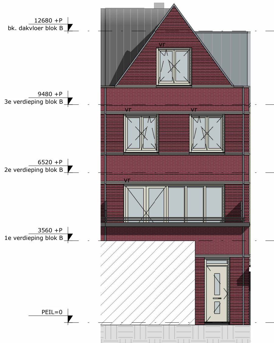
VOORGEVEL Stadsplein zuid
