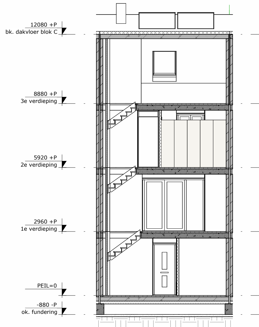
DWARSDOORSNEDE
