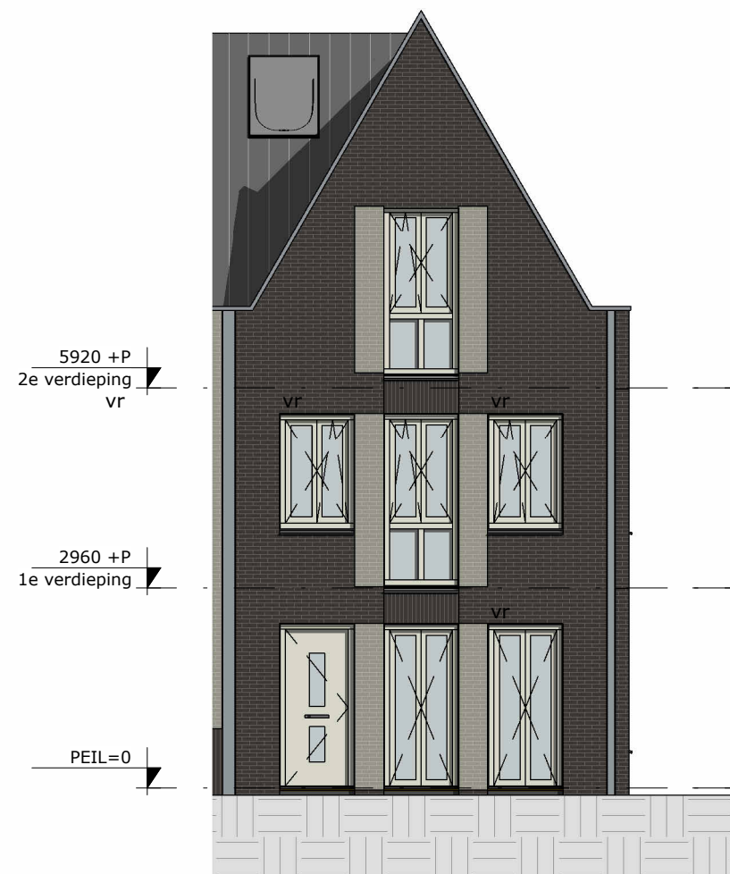
VOORGEVEL
