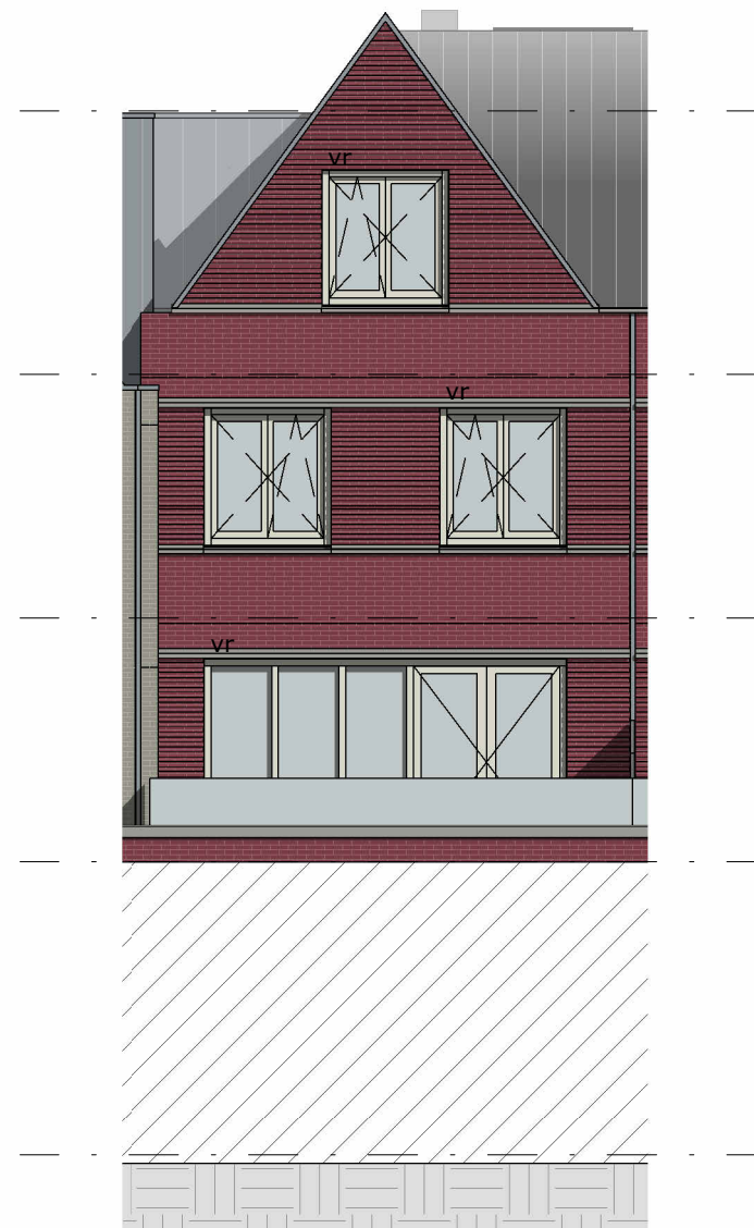
ACHTERGEVEL IJsselmeerzijde noord
