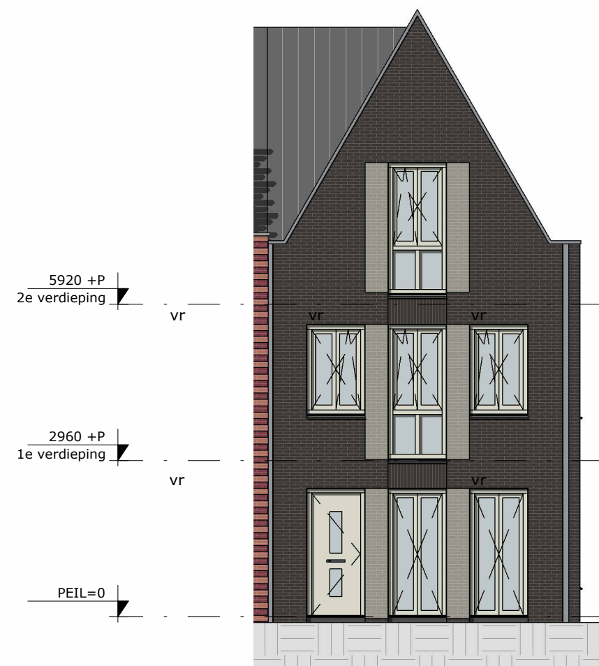
VOORGEVEL
