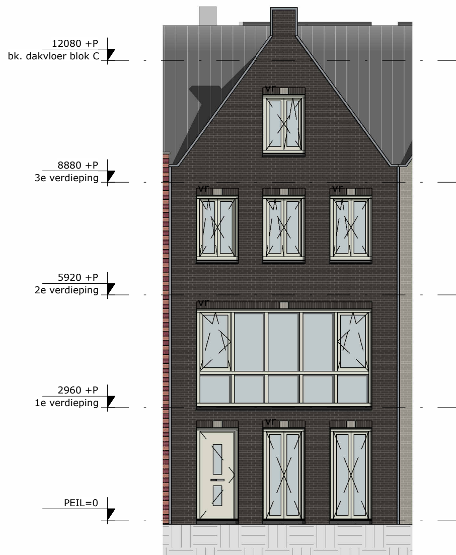
VOORGEVEL IJsselmeerzijde noord
