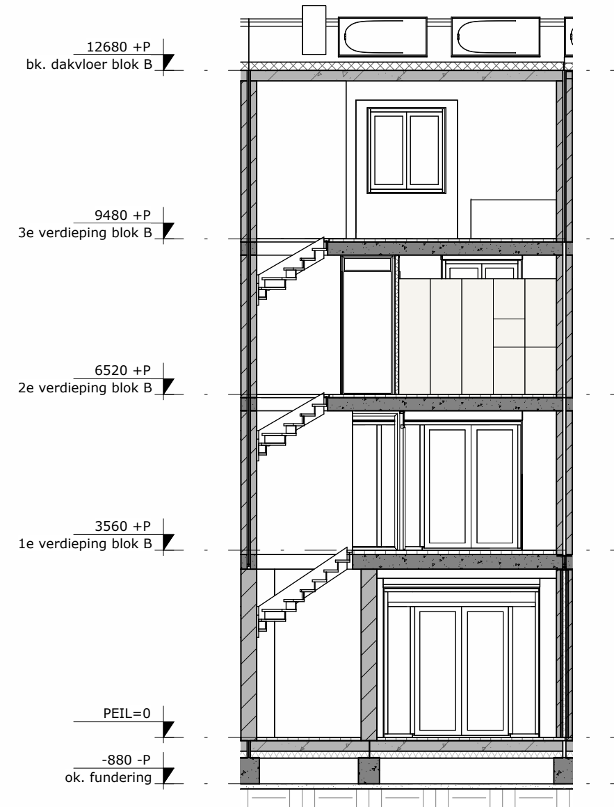
DWARSDOORSNEDE
