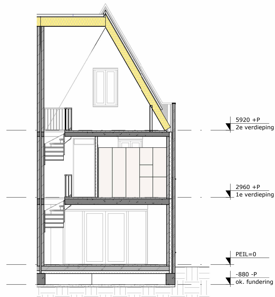
DWARSDOORSNEDE
