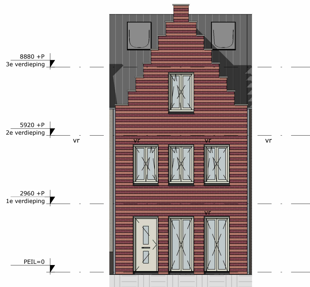
VOORGEVEL
