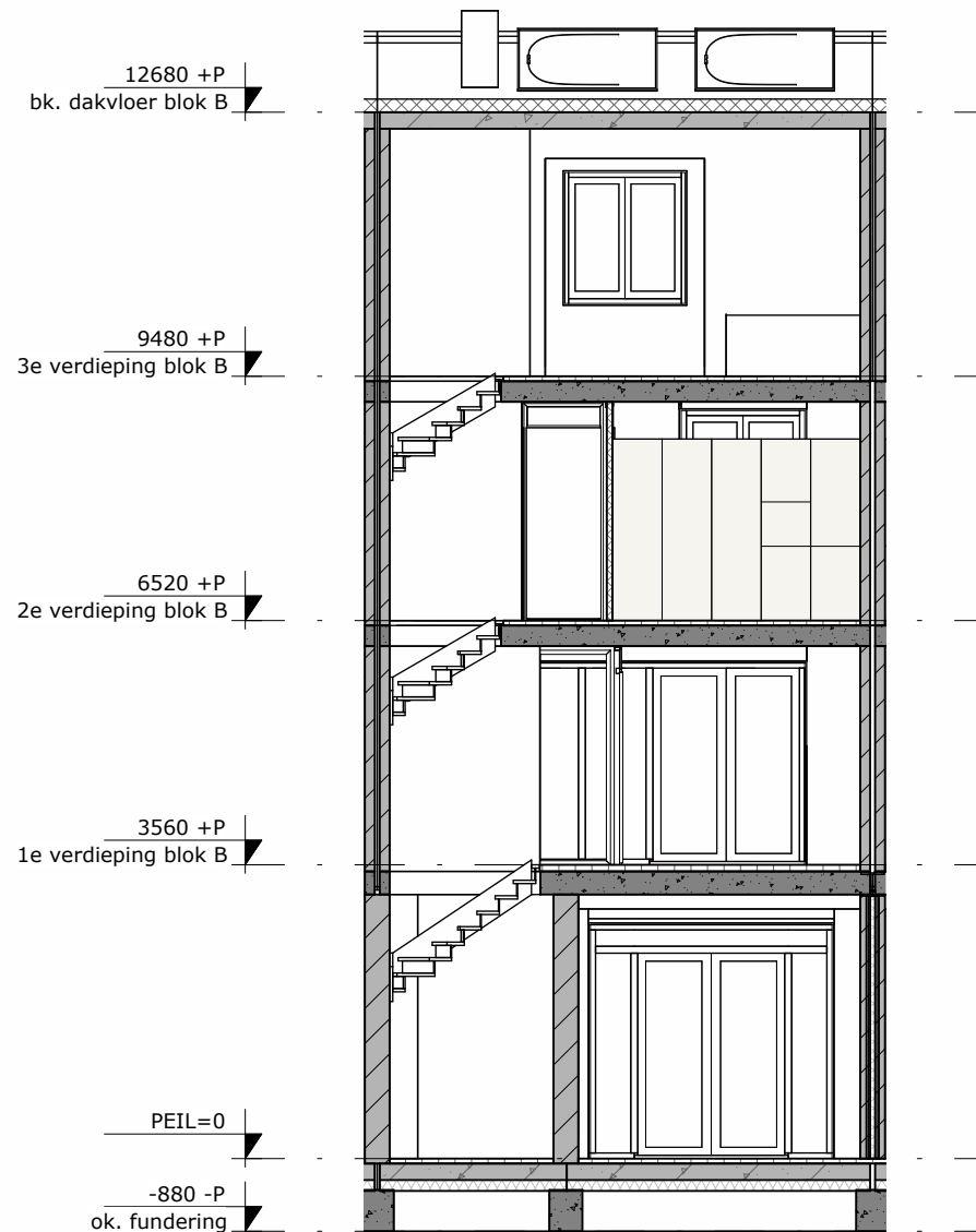
DWARSDOORSNEDE
