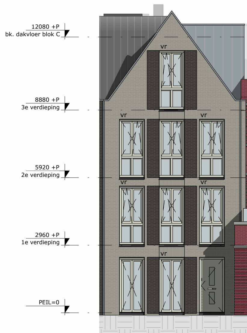
VOORGEVEL IJsselmeerzijde noord
