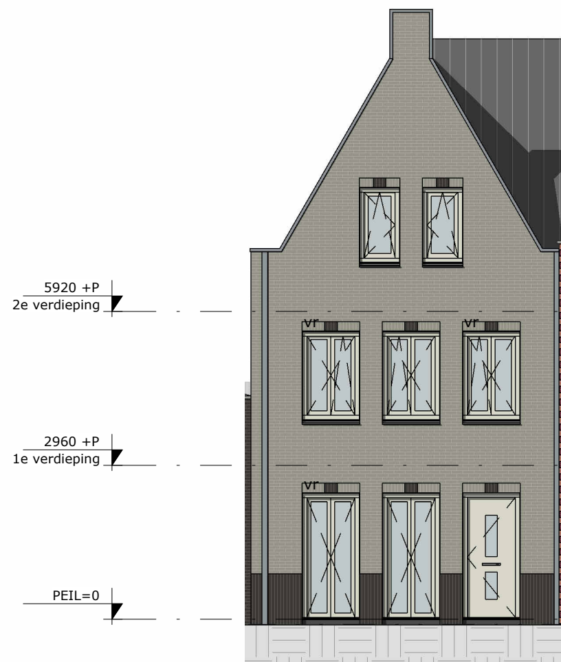
VOORGEVEL
