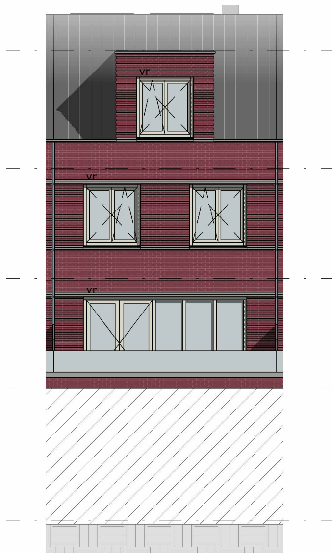
ACHTERGEVEL IJsselmeerzijde noord
