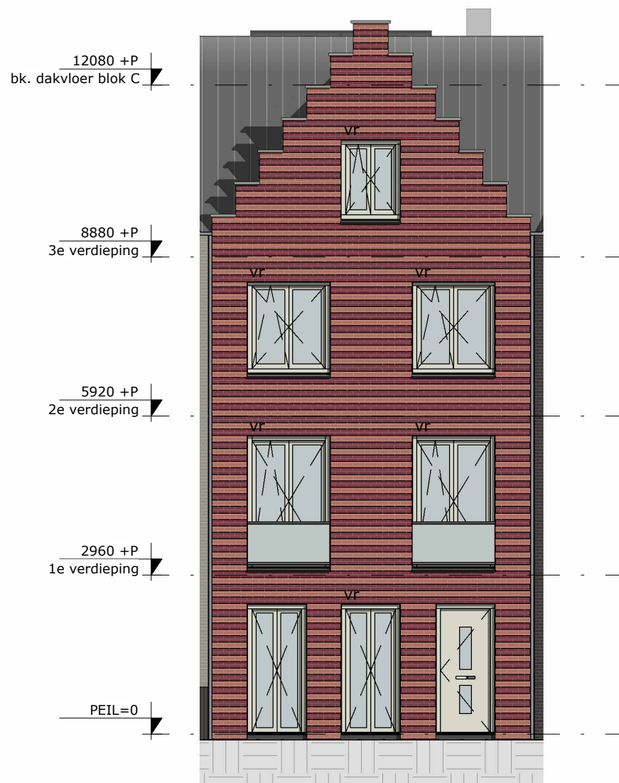
VOORGEVEL IJsselmeerzijde noord
