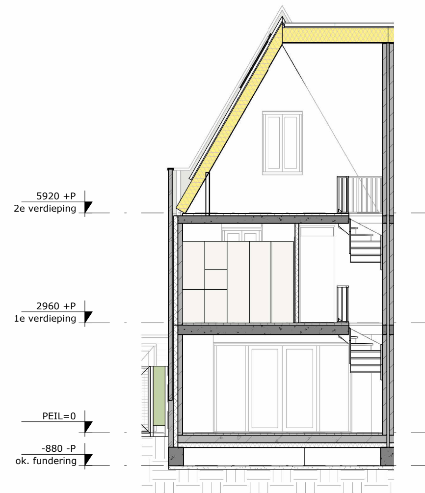
DWARSDOORSNEDE
