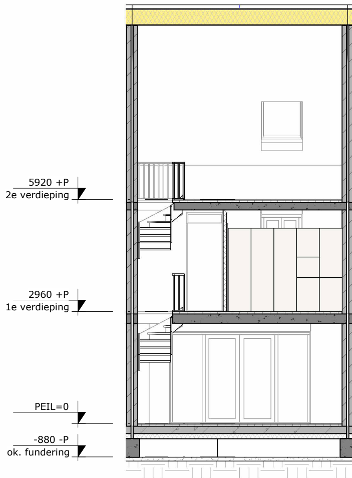
DWARSDOORSNEDE
