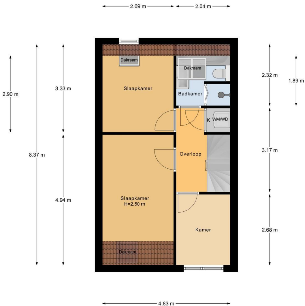
1e Verdieping
