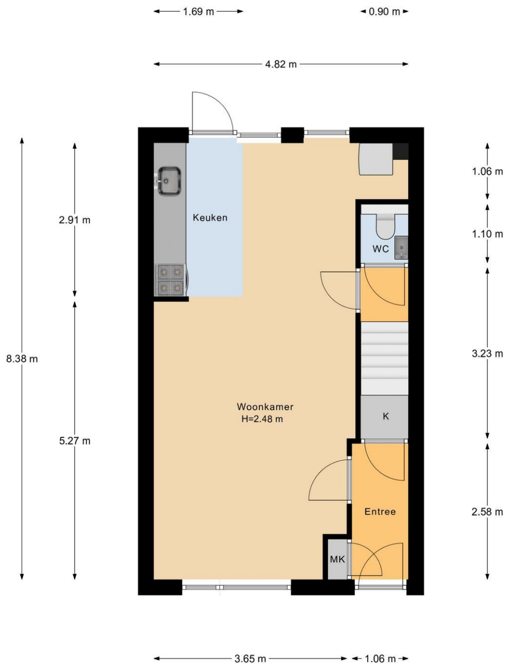
Begane Grond
