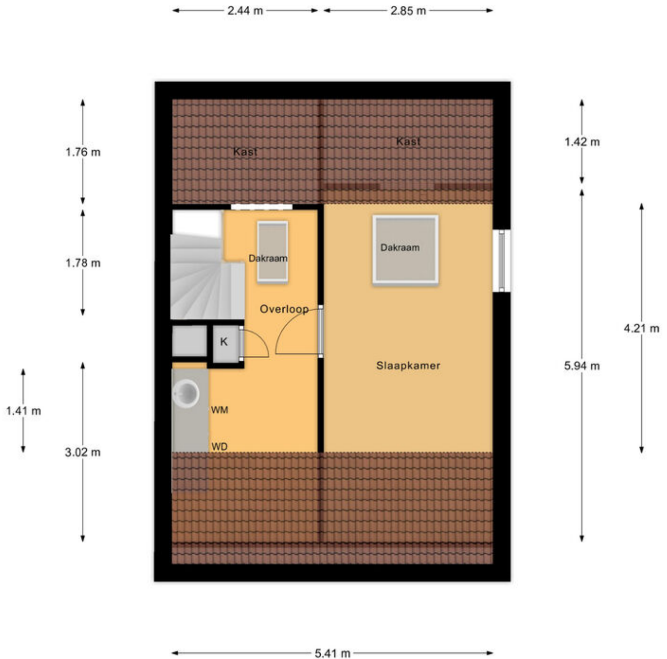
2e Verdieping
