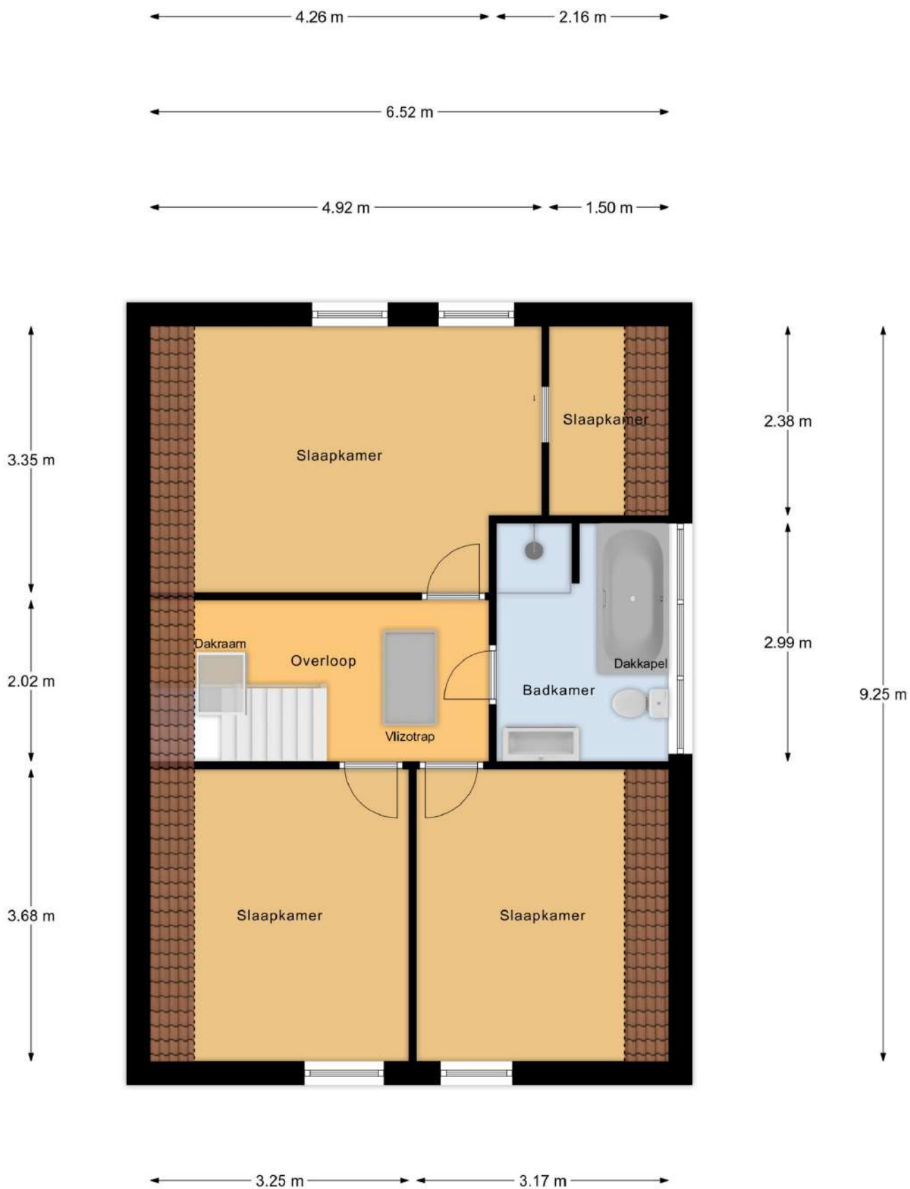
1e Verdieping
