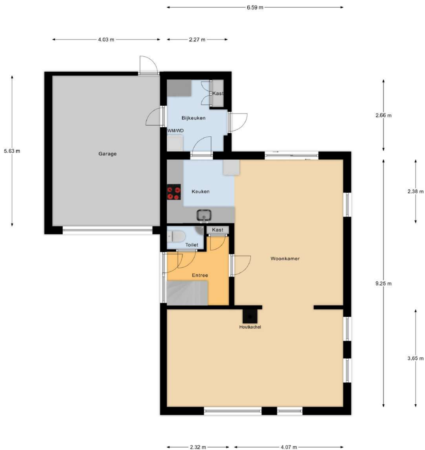
Begane Grond
