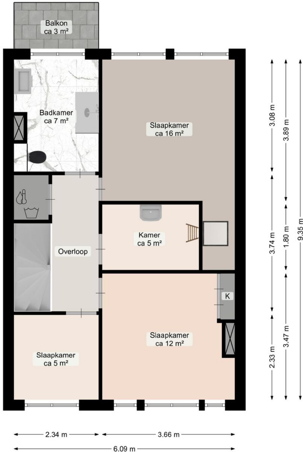
Tweede verdieping
