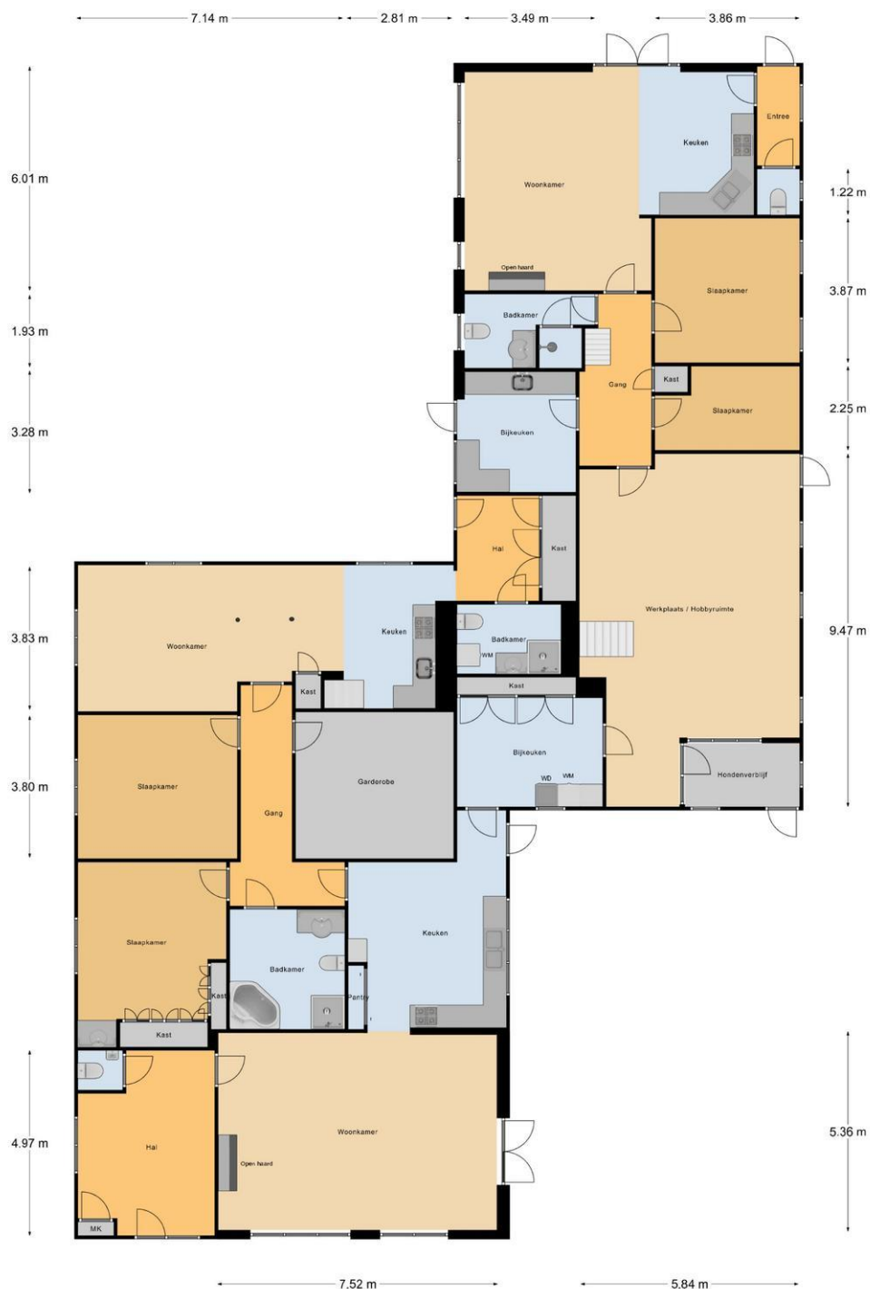
Begane Grond
