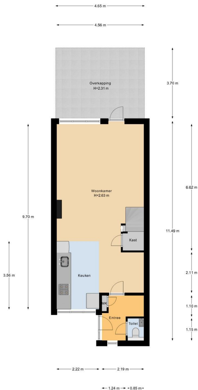
Begane Grond
