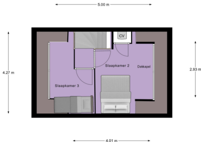
Voorstel 4: Tweede Verdieping 2 slaapkamers Aan deze tekening kunnen geen rechten ontleend worden.
