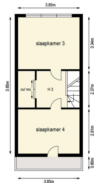
tweede verdieping
