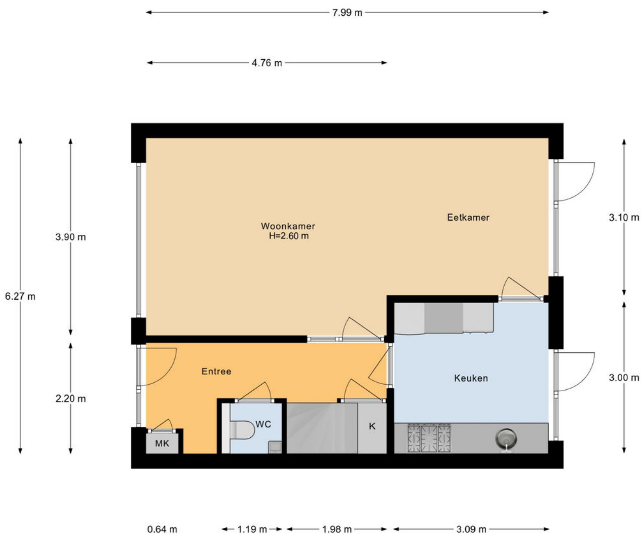
Begane Grond
