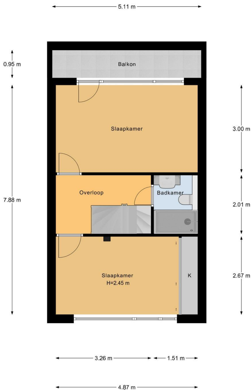
1e Verdieping
