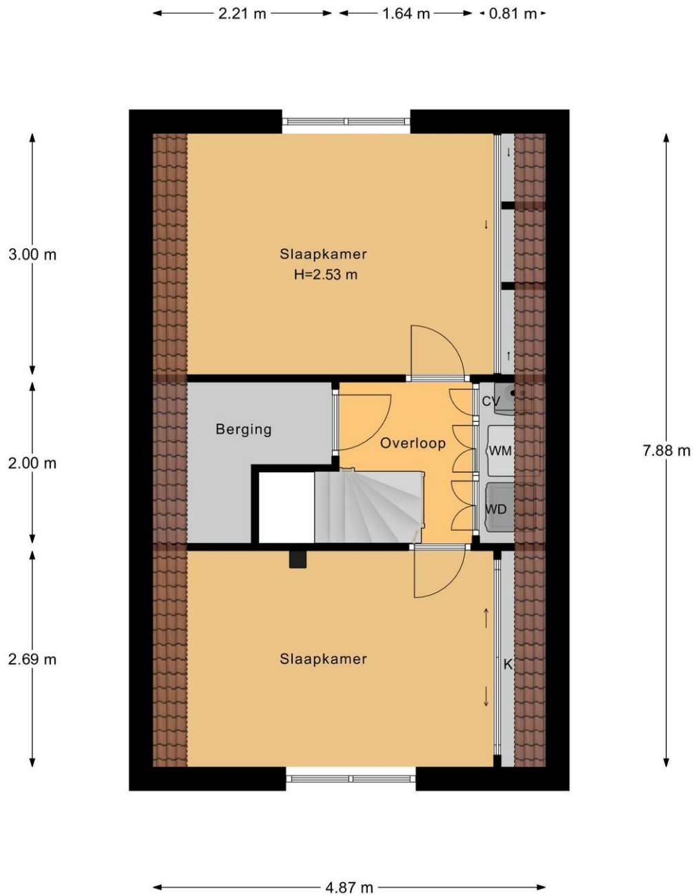
2e Verdieping
