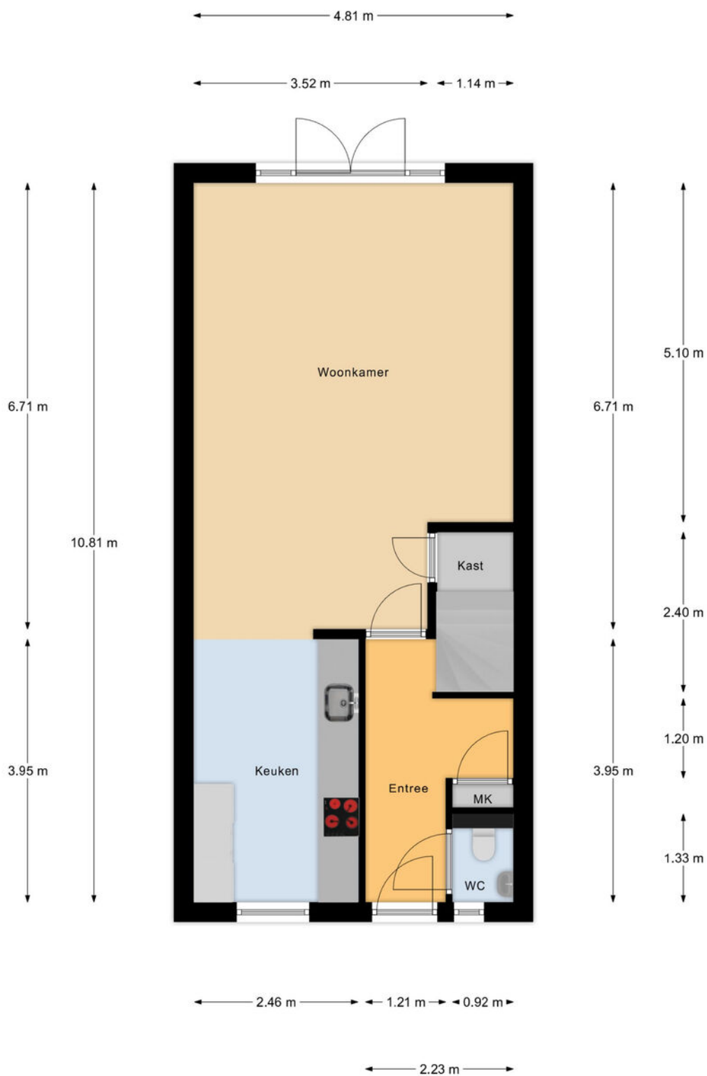
Begane Grond
