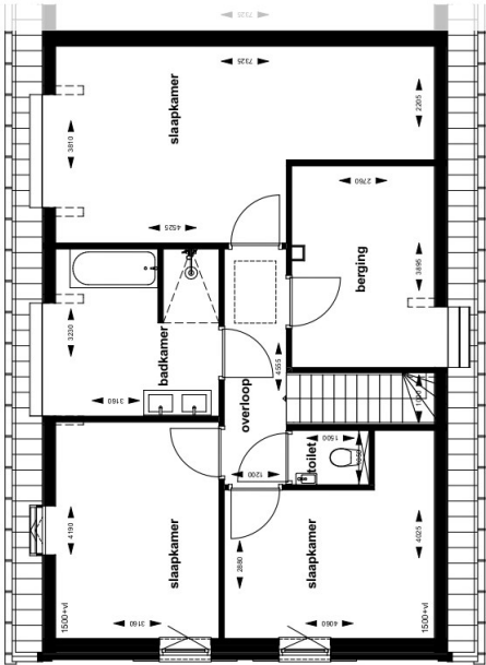
1e verdieping 1:100
