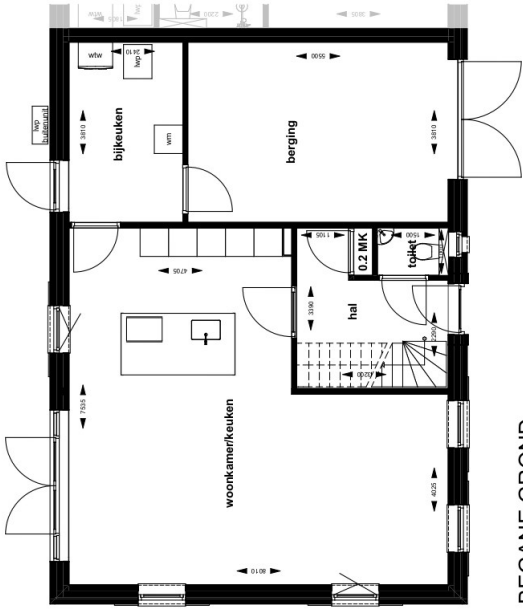
BEGANE GROND 1:100
