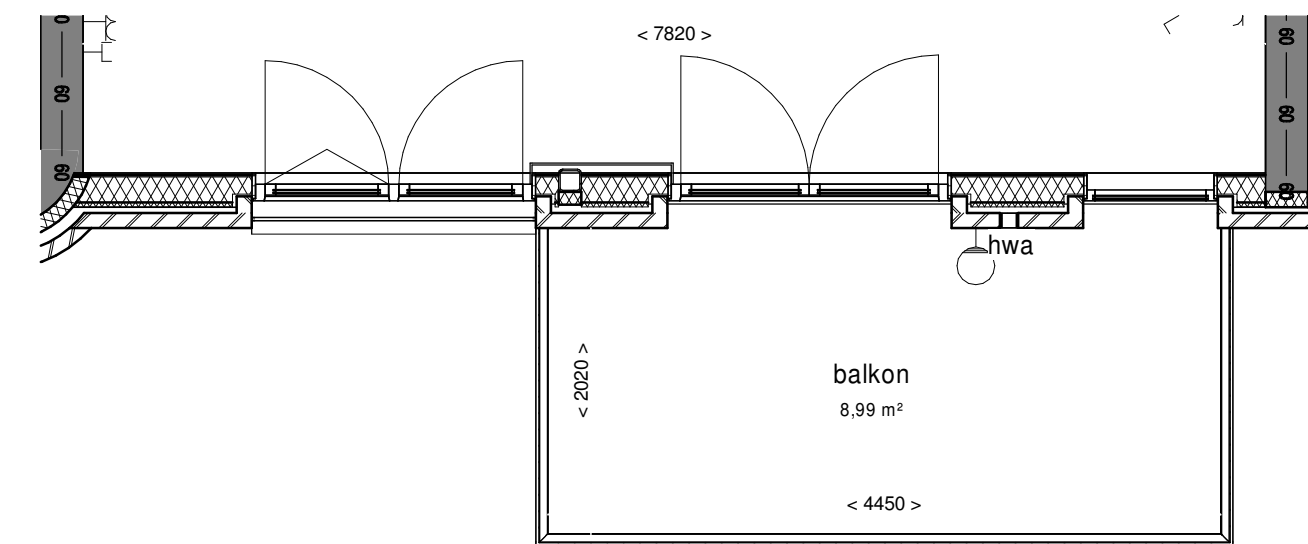
westgevel Bouwnrs.: 03.20/05.15
