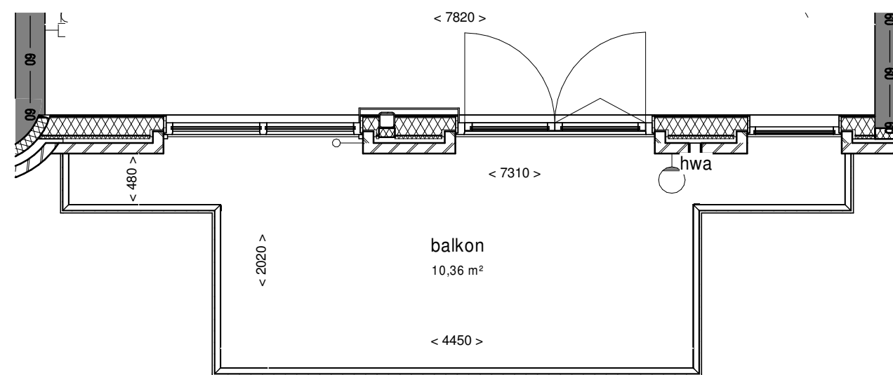
westgevel Bouwnrs.: 02.20/04.20
