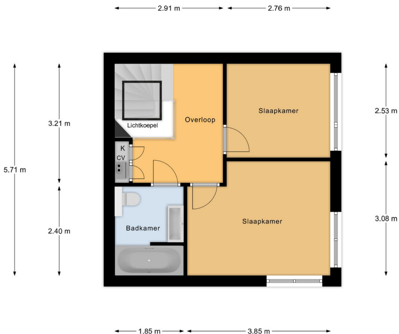
1e Verdieping
