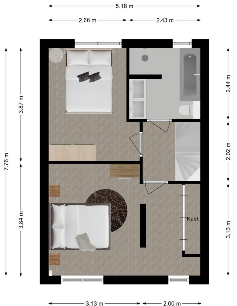
Plattegrond eerste verdieping Aan deze tekening kunnen geen rechten worden ontleend
