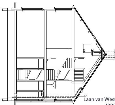
Doorsnede
