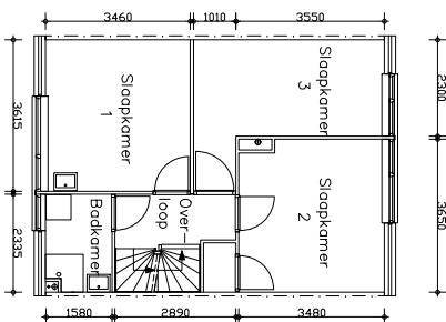
Verdieping
