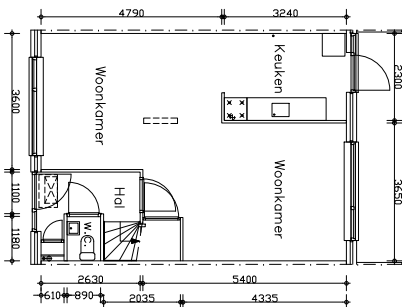
Beganegrond
