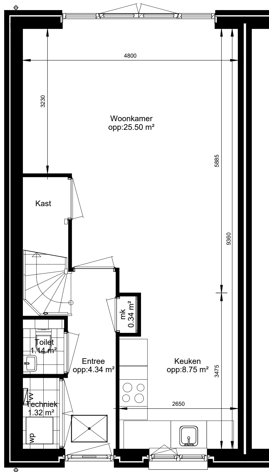
BEGANE GROND
