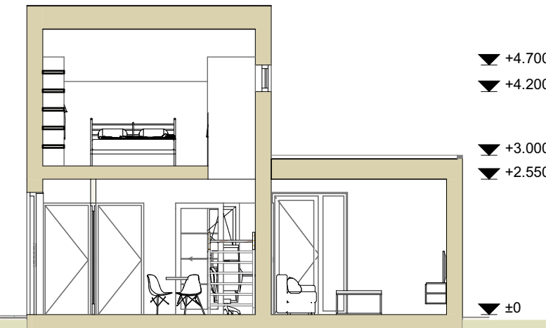
doorsnede B-B
