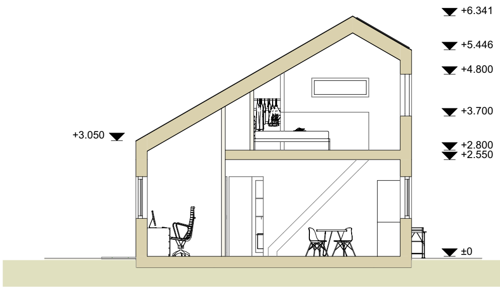
doorsnede A-A
