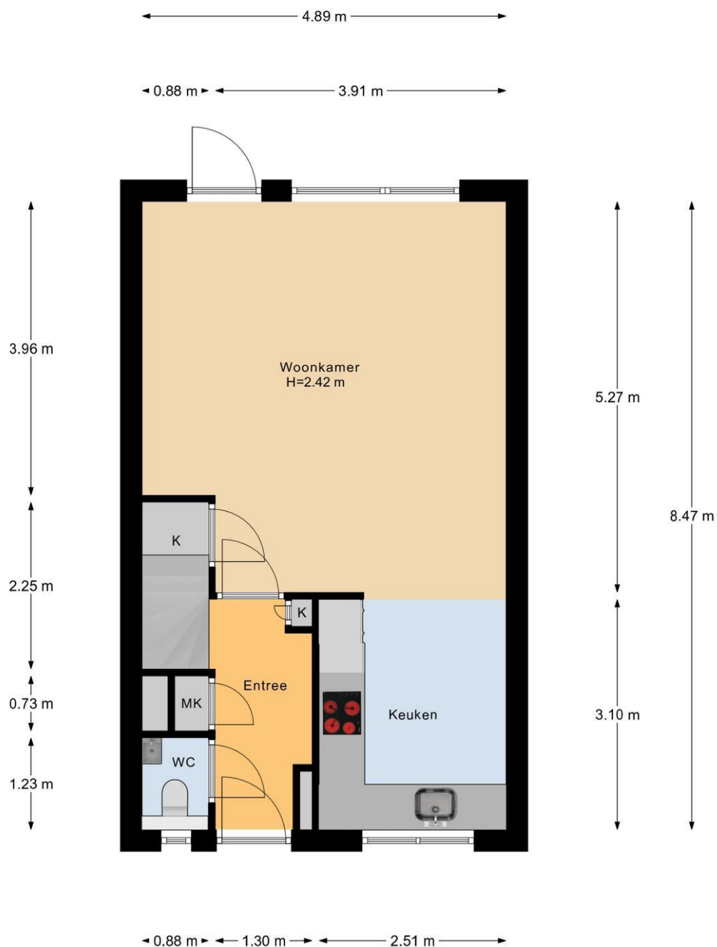
Begane Grond
