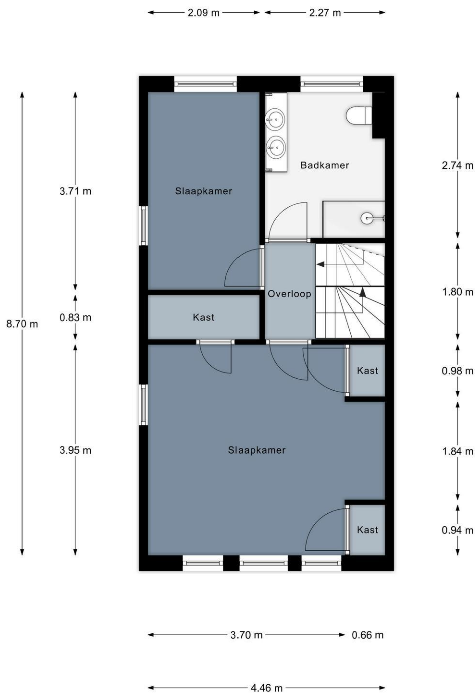
Eerste Verdieping
