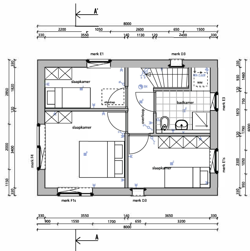
VERDIEPING
