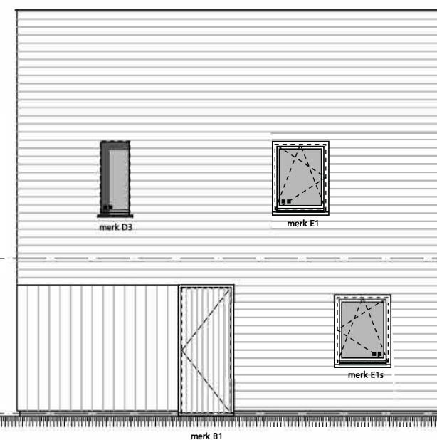
ACHTERGEVEL
