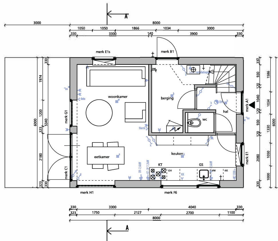
BEGANE GROND
