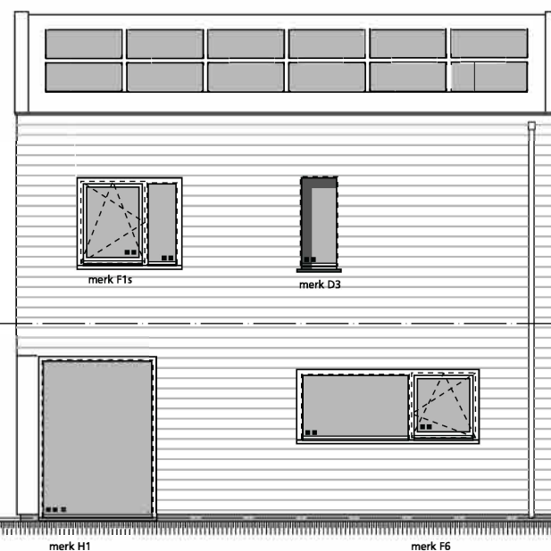
ZONGEVEL
