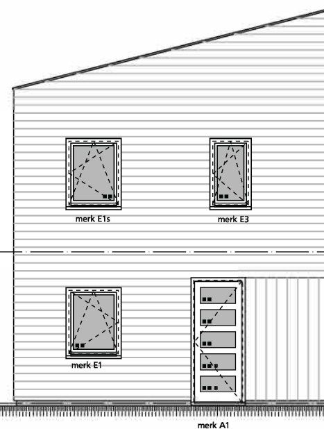
STRAATGEVEL
