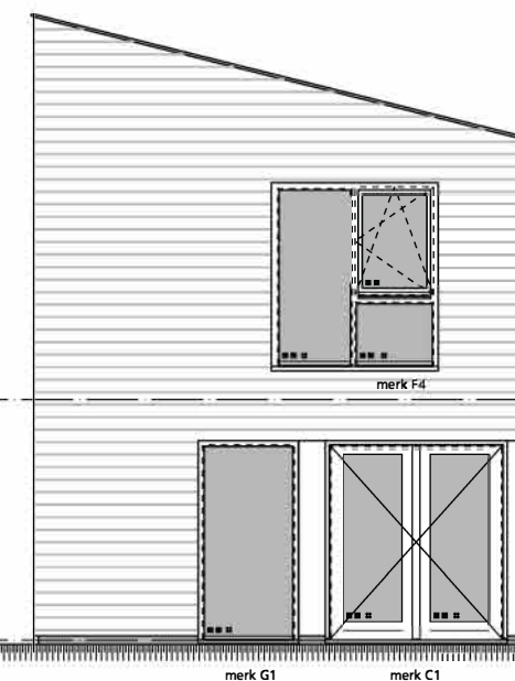
TUINGEVEL
